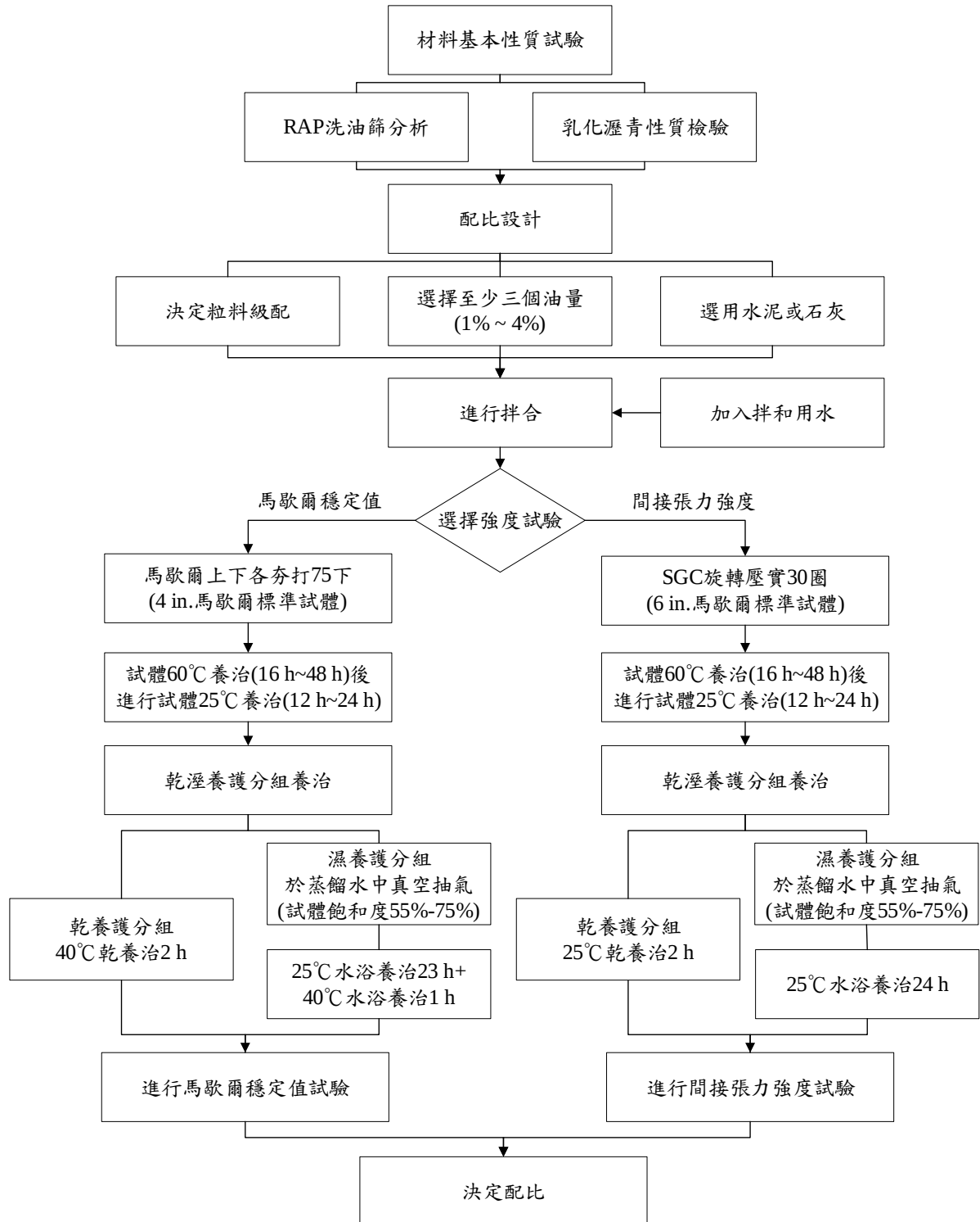
圖 1 冷拌再生乳化瀝青混凝土配合設計流程圖
