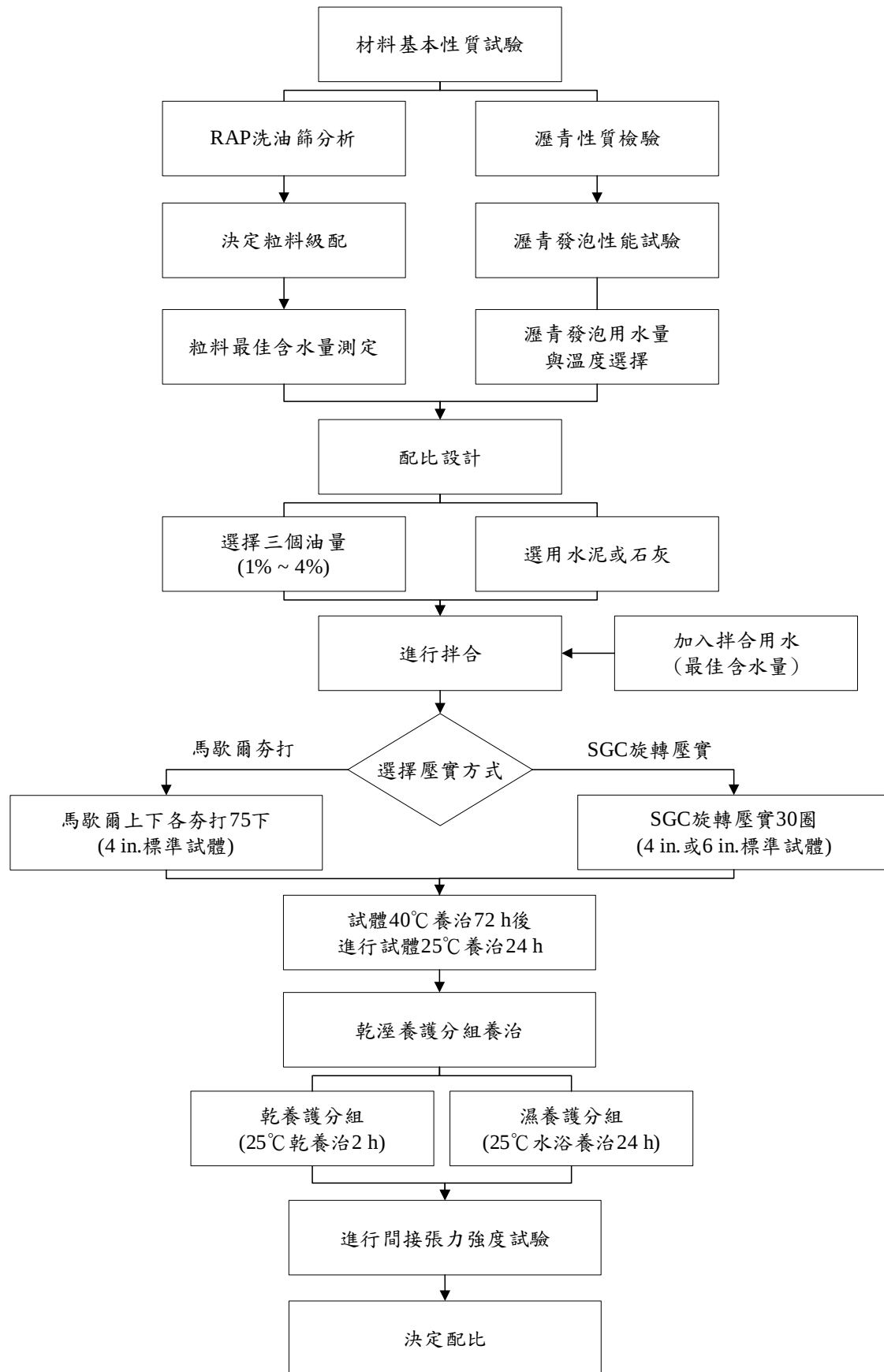
圖 1 冷拌再生發泡瀝青混凝土配合設計流程圖
