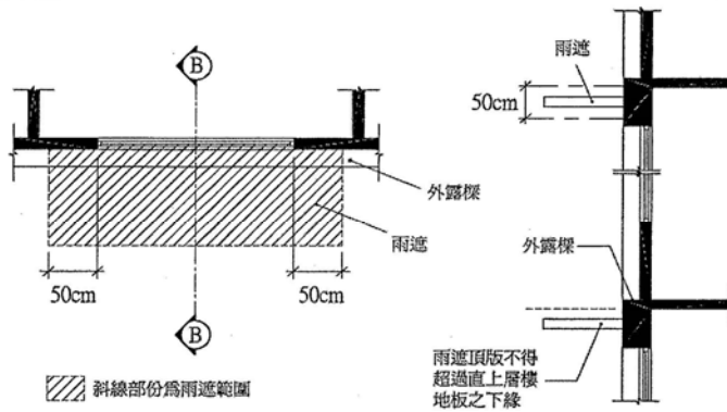
B-B 平面圖
