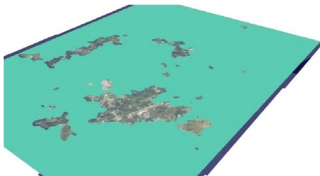
模擬海水面上升 10 m
