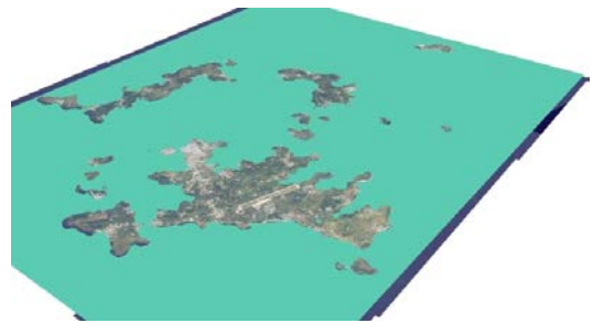
模擬海水面上升 5 m
