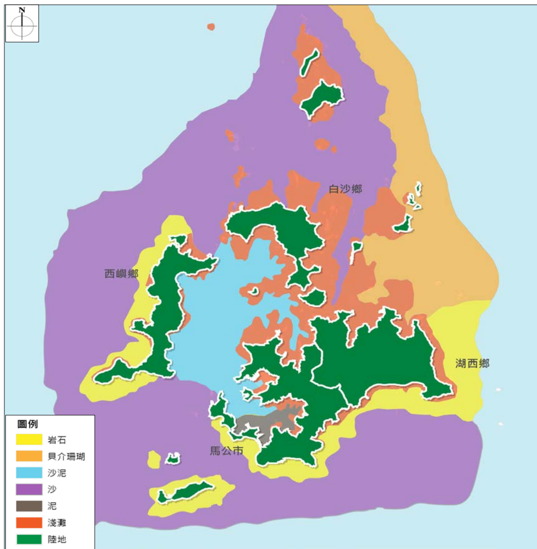
圖2-7 澎湖縣近海海底底質圖
