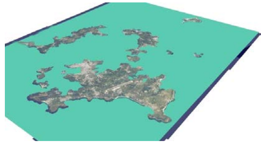
模擬海水面上升 1 m
