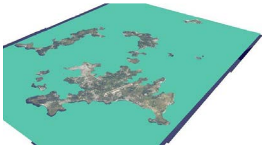
模擬海水面上升 3 m
