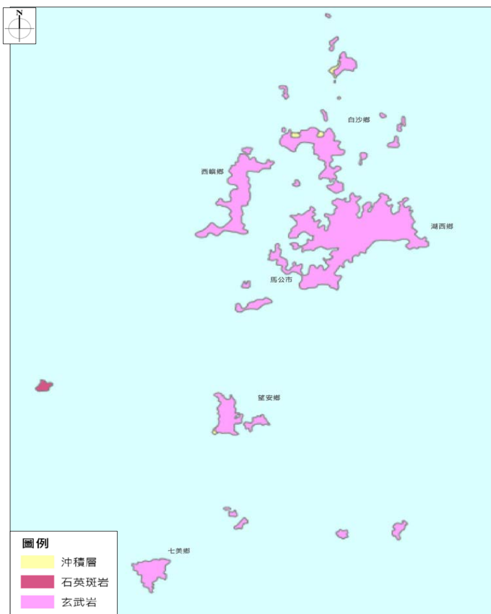
圖2-2 澎湖縣地質結構分布示意圖
