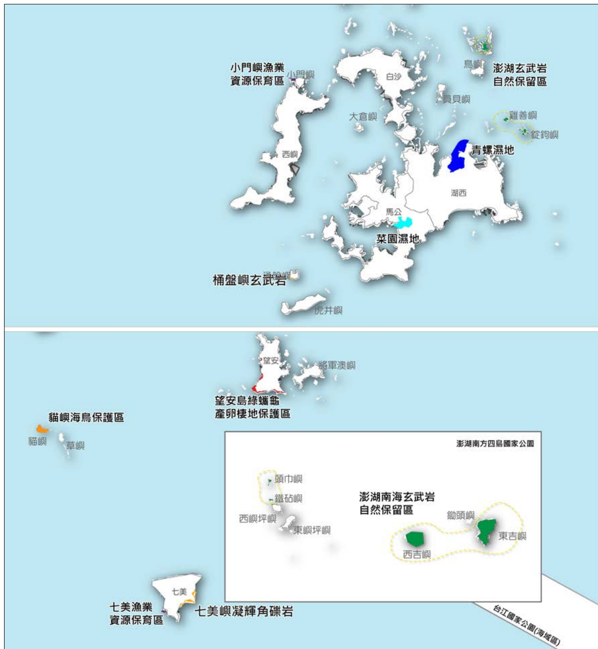
圖2-10 澎湖縣自然生態分佈示意圖
