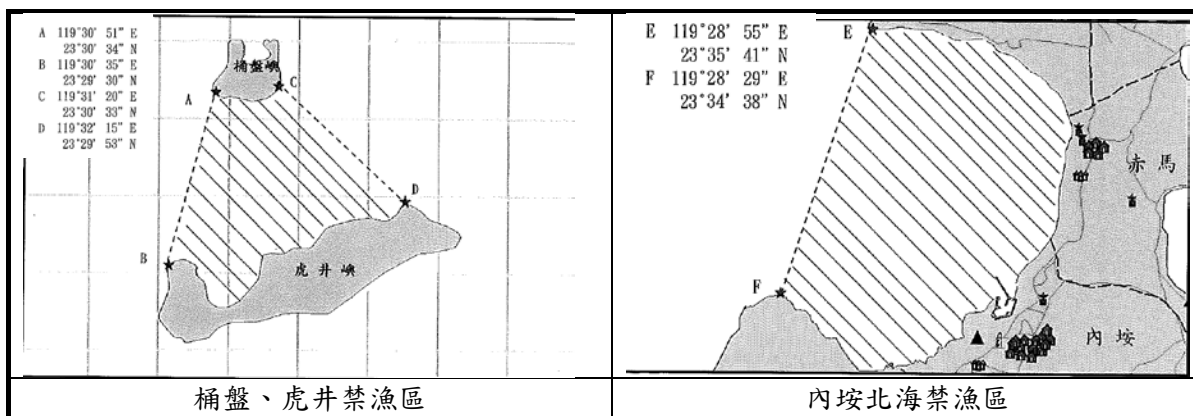
圖2-23 桶盤、虎井、內垵北海海域禁漁區區位圖
