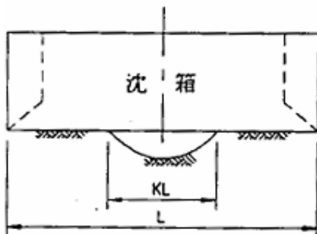
圖-解 6.7-1 簡支承狀況
