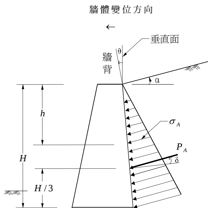
圖 7.1 主動土壓力圖
