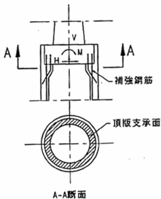
圖-解 6.7-13 錨碇鋼筋
