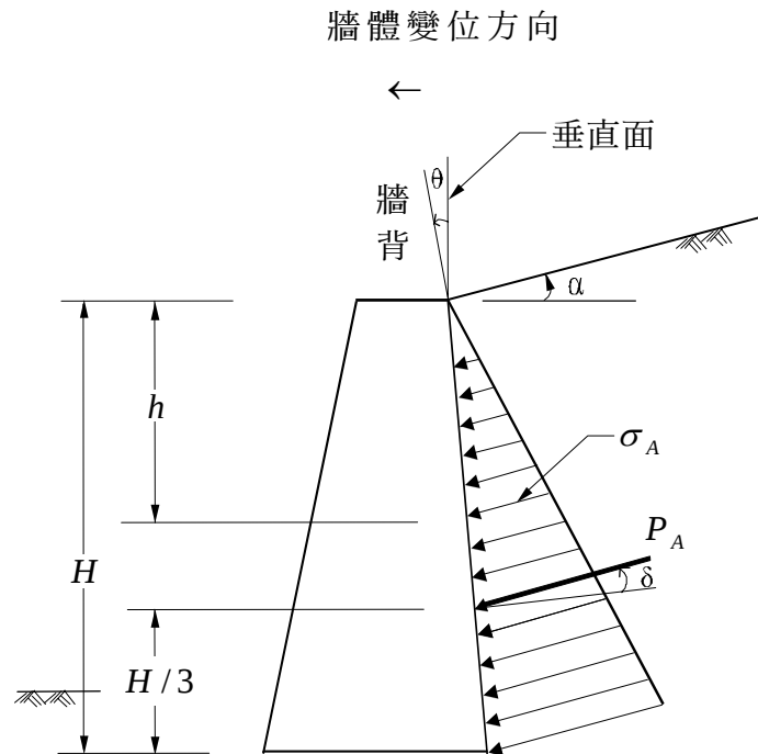
圖 7.3-1 主動土壓力圖
