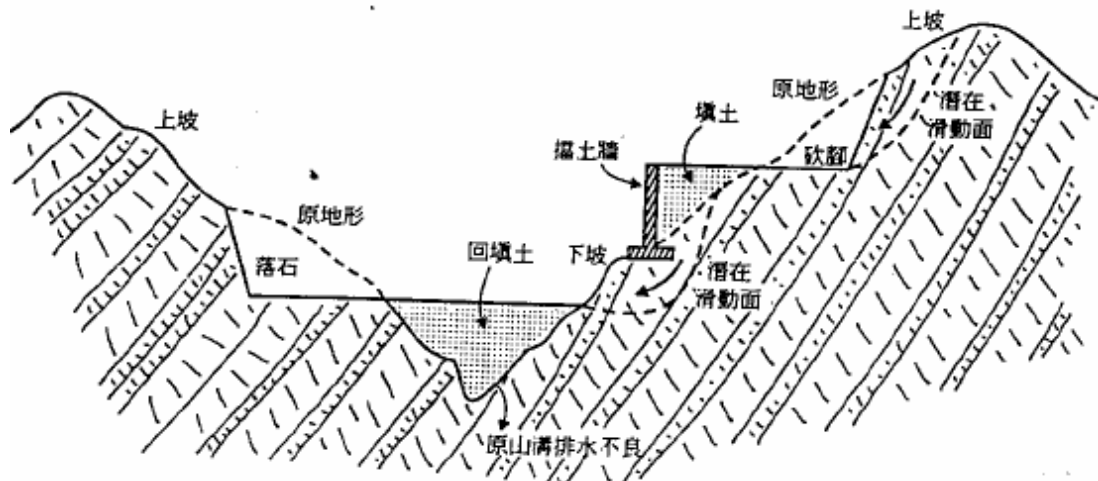
圖-解 3.1-1 山坡地整地工程可能引起之邊坡穩定問題
