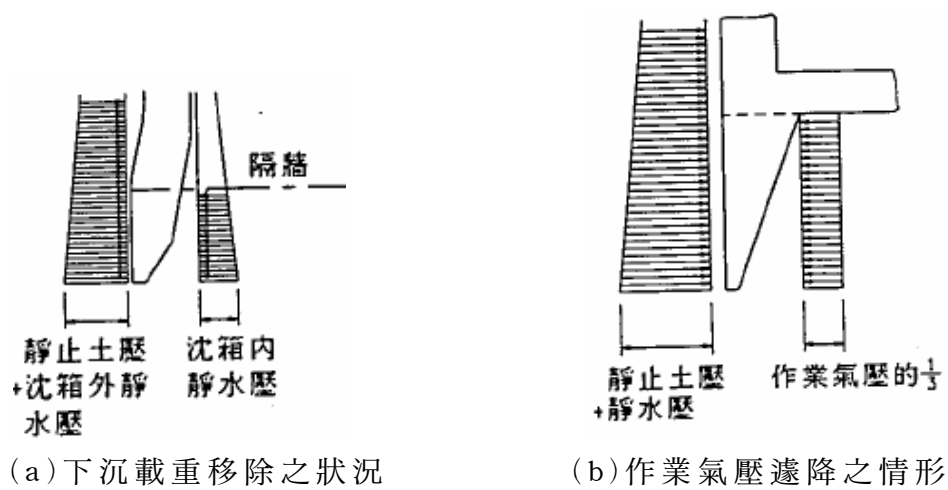
圖-解 6.7-16 刃口之設計載重
