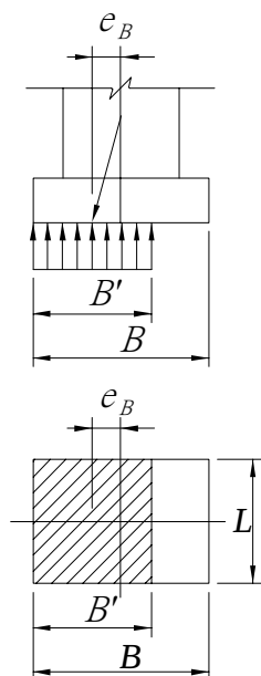
(a) 單向偏心作用
