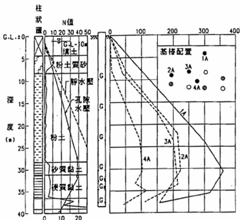
圖-解 5.3-11 群樁對負摩擦力之影響
