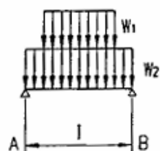
載重圖
