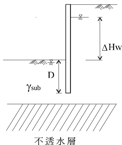
圖8.8-3 砂湧檢討
