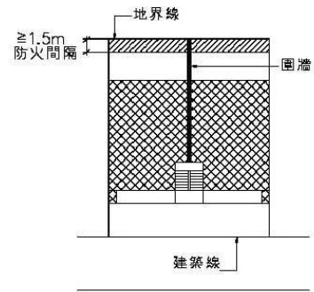
第110條 圖110-(3)
