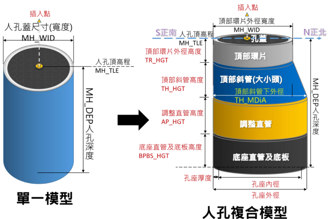
圖 1.2 污水下水道人孔 3D 模型示意圖
