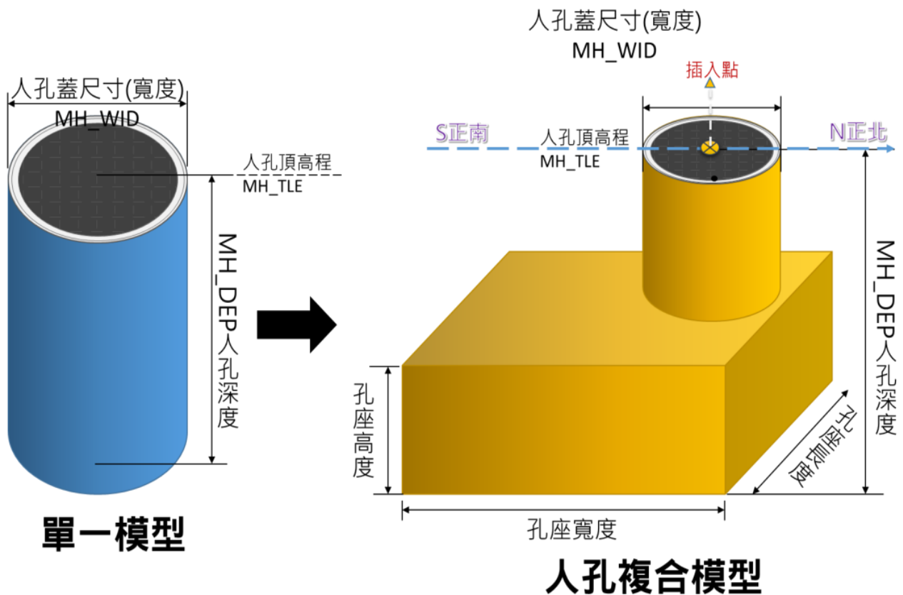
圖 1.1 雨水下水道人孔 3D 模型示意圖
