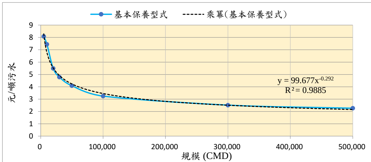
圖 2.2-2 基本保養型式之單位處理費用迴歸分析
