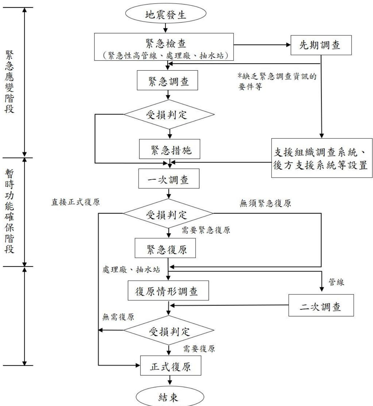
圖 3.7-4 地震緊急應變處理及災後復原流程（例）
