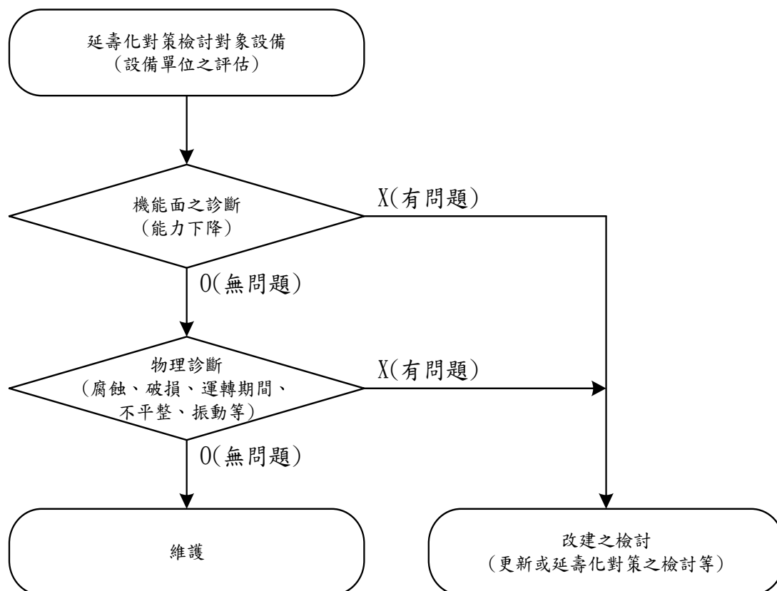
圖 6.6-9 健全度評估流程例（延壽化對策檢討對象設備之設備單位評價）
