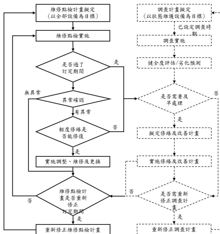
圖 6.4-1 維護點檢執行步驟（時間計畫維護之機械電氣設備）
