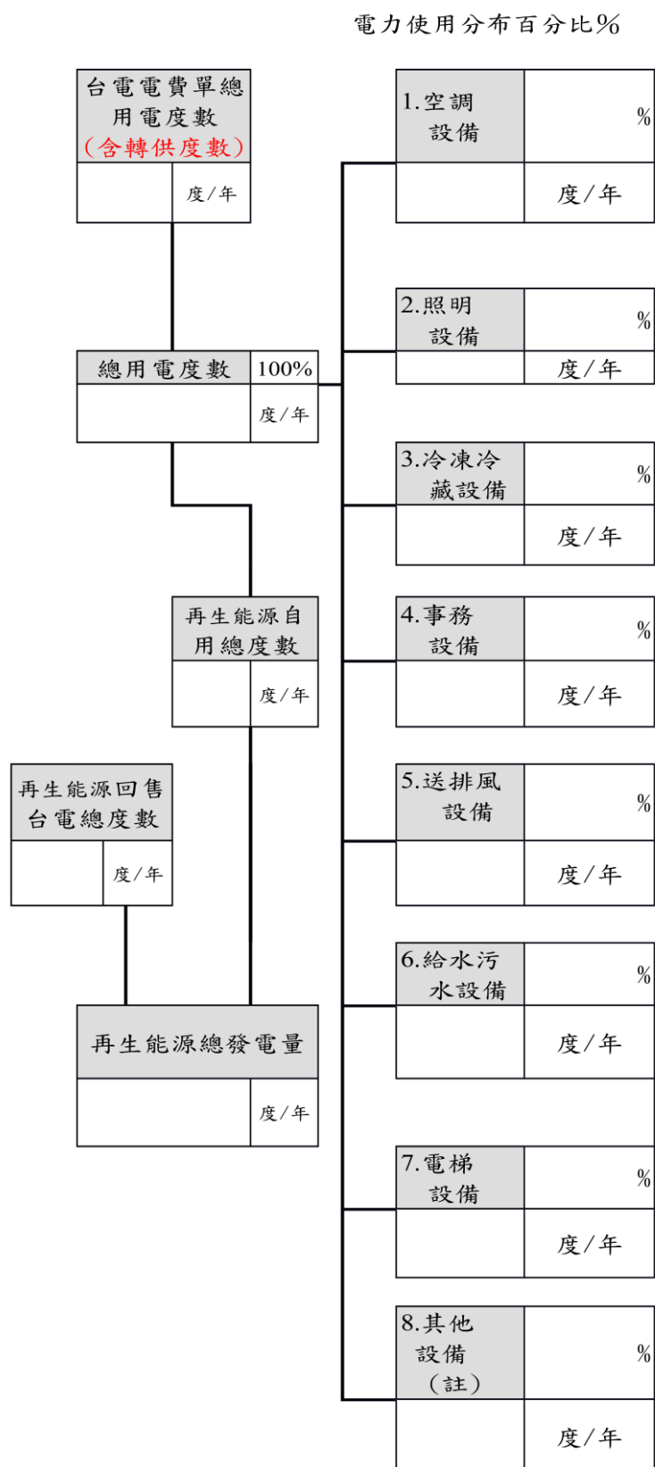
圖 3.6-3 能源流程分析-電能用量平衡圖（例）
