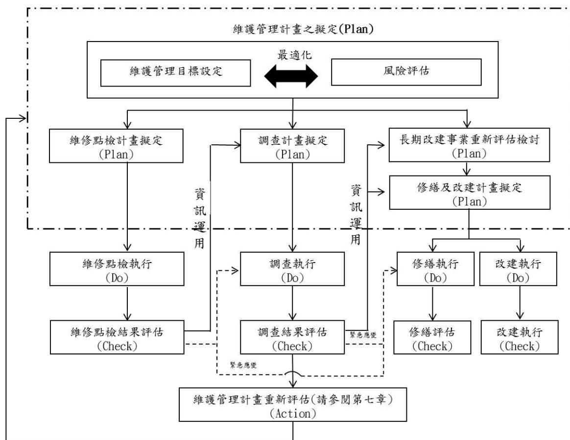
圖 6.1-1 雨水抽水站計畫性維護管理執行步驟
