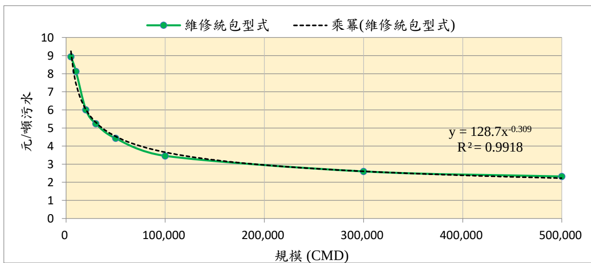
圖 2.2-4 維修統包型式之單位處理費用迴歸分析
