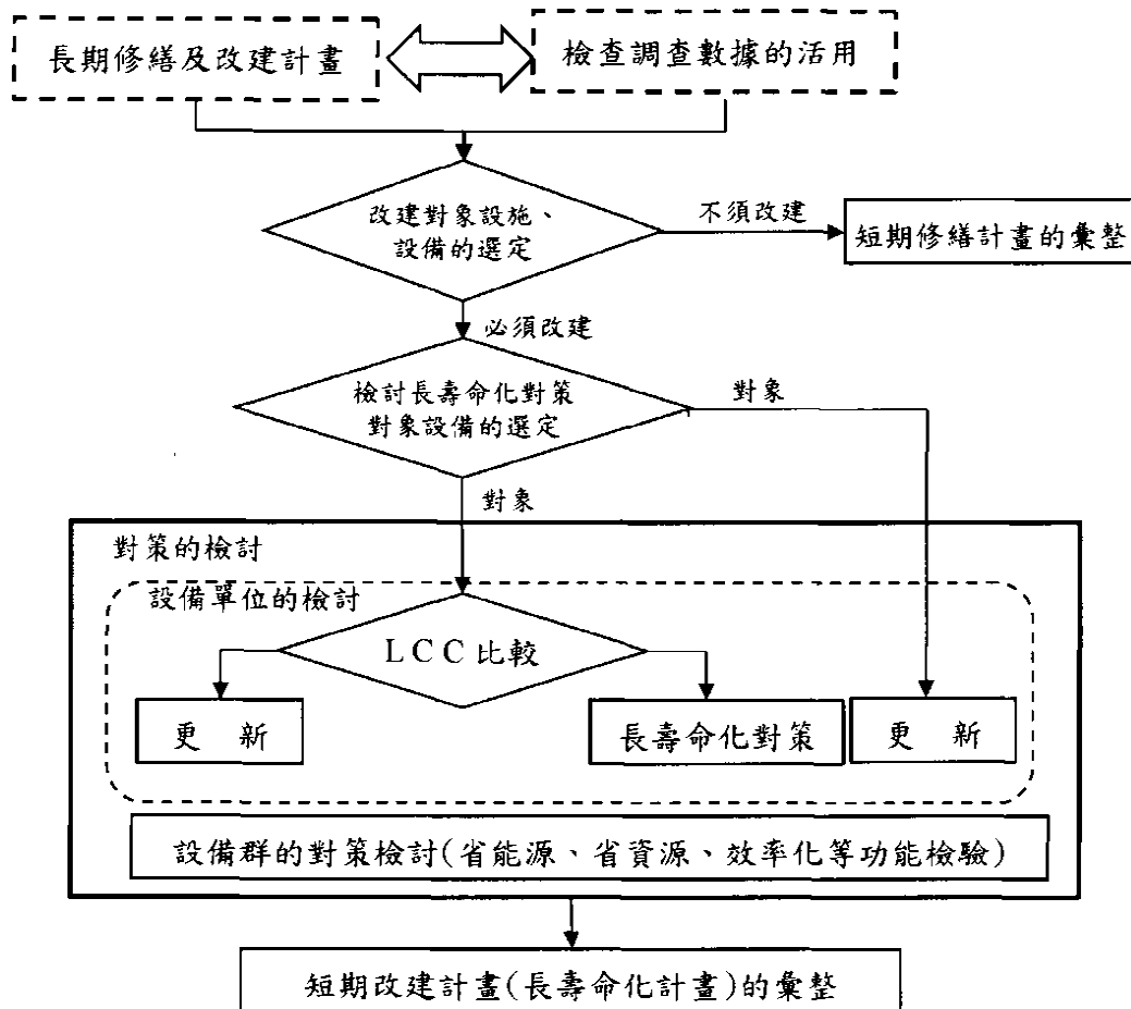
圖 6.6-3 短期修繕及重置計畫之擬定流程（例）
