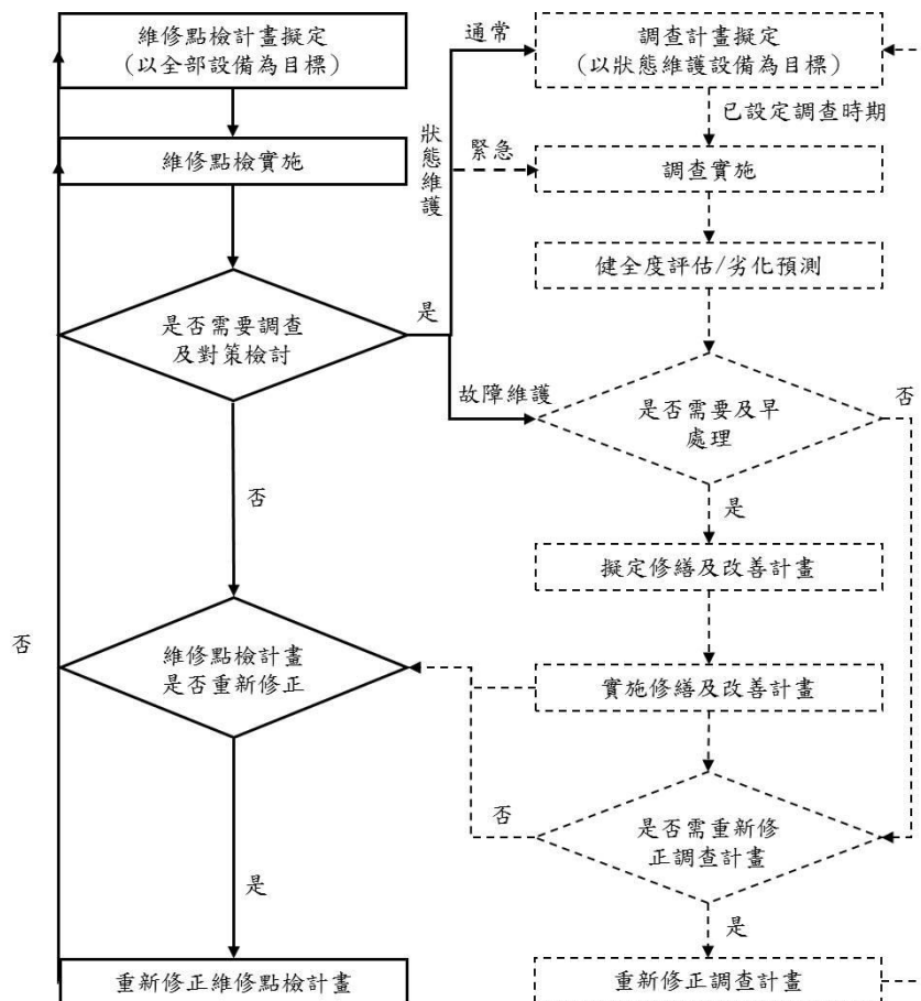
圖 6.4-2 維護點檢執行步驟（狀態維護及故障維護之機械電氣設備）
