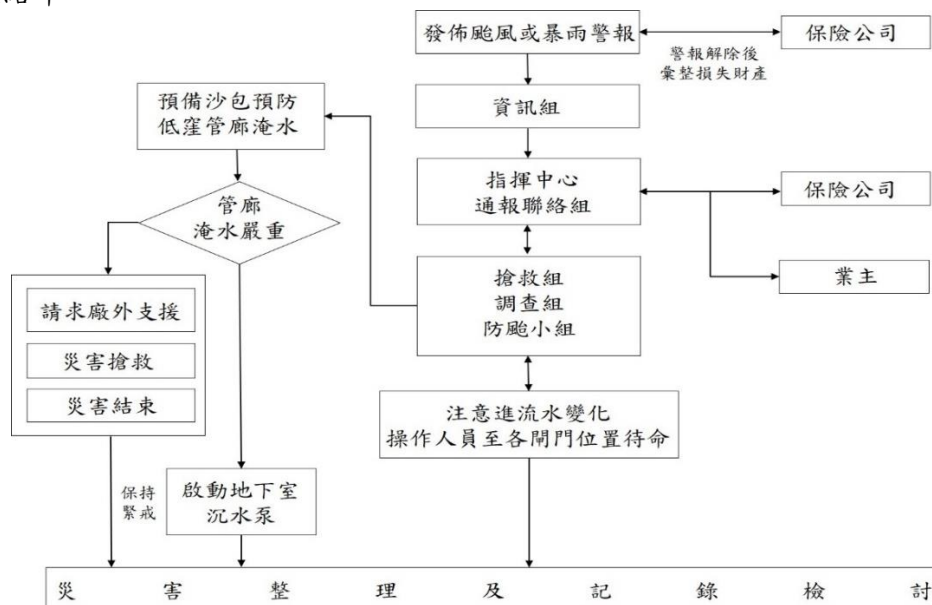
圖 3.7-3 暴雨、颱風之緊急應變程序（例）
