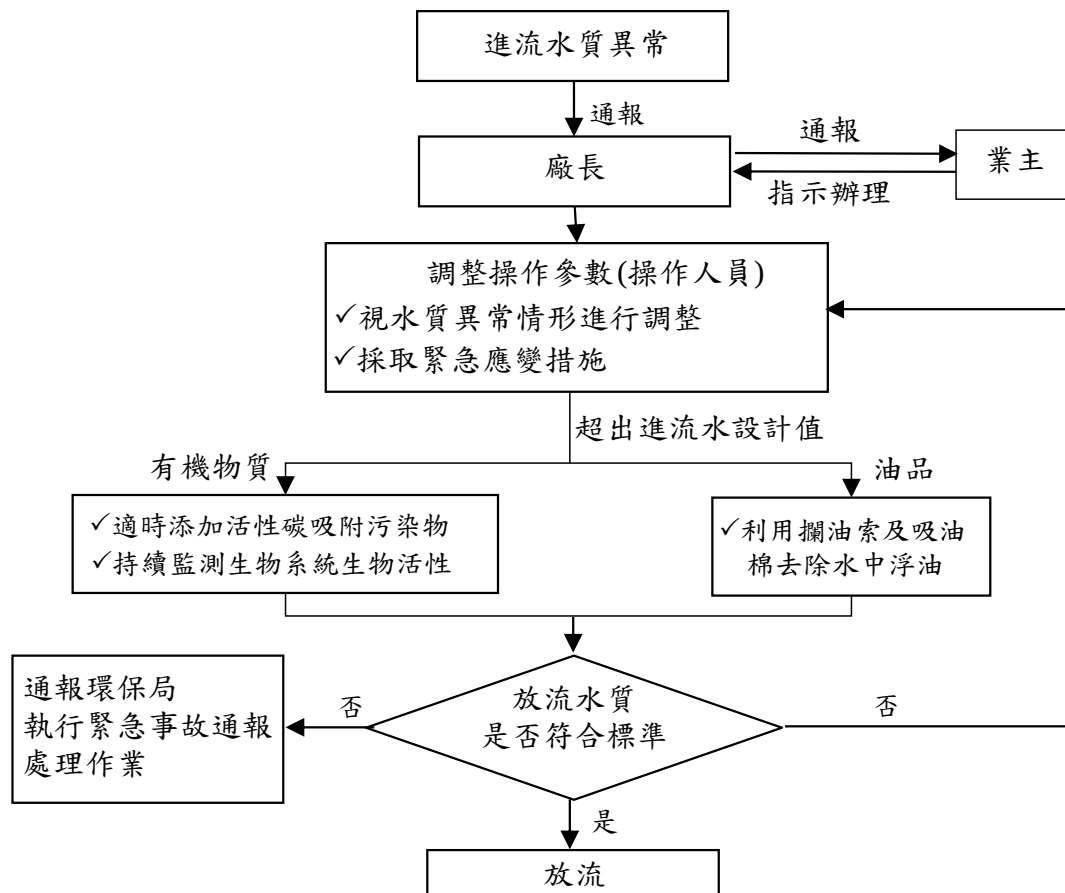
圖 3.7-6 進流水質異常應變流程（例）
