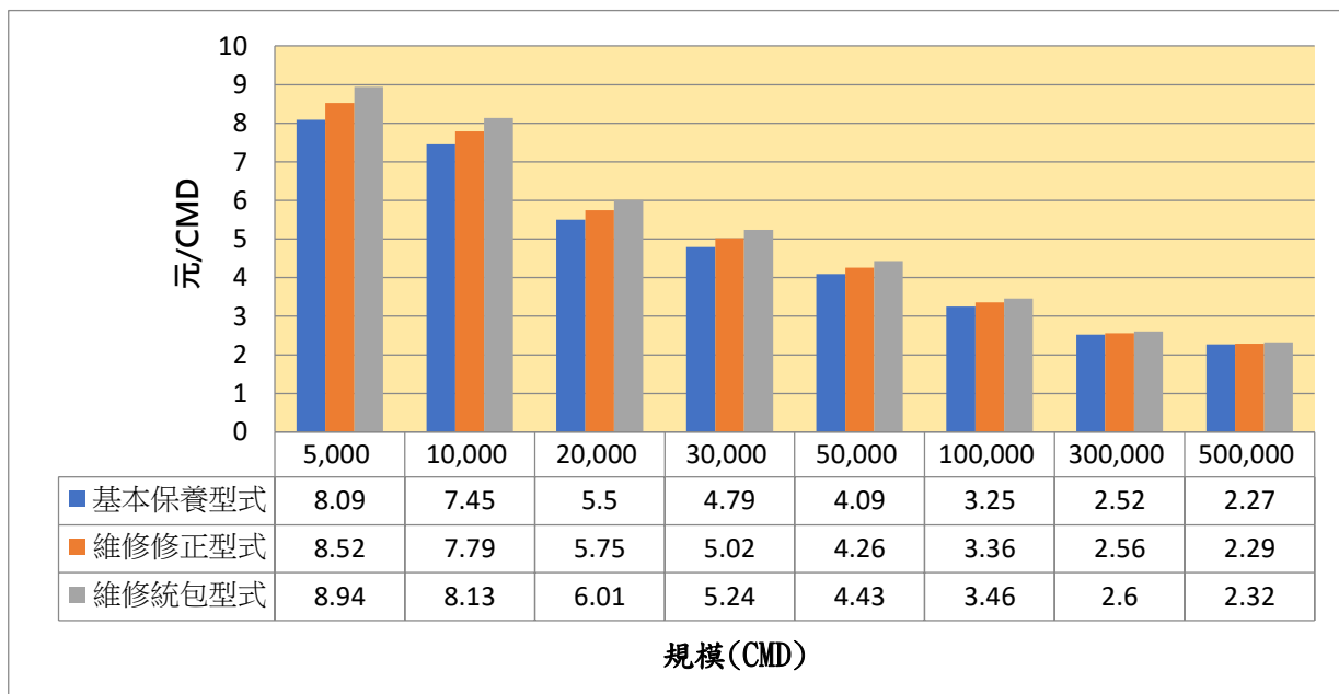
圖 2.2-1 不同維護型式依不同處理規模之單位處理費用
