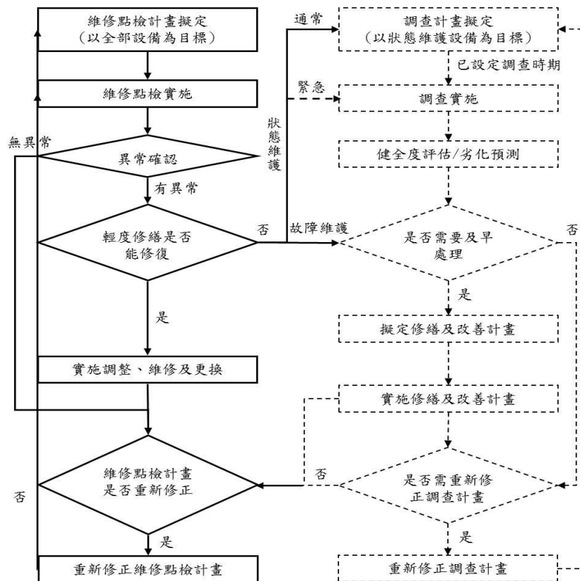
圖 6.4-2 維護點檢執行步驟（狀態維護及故障維護之機械電氣設備）
