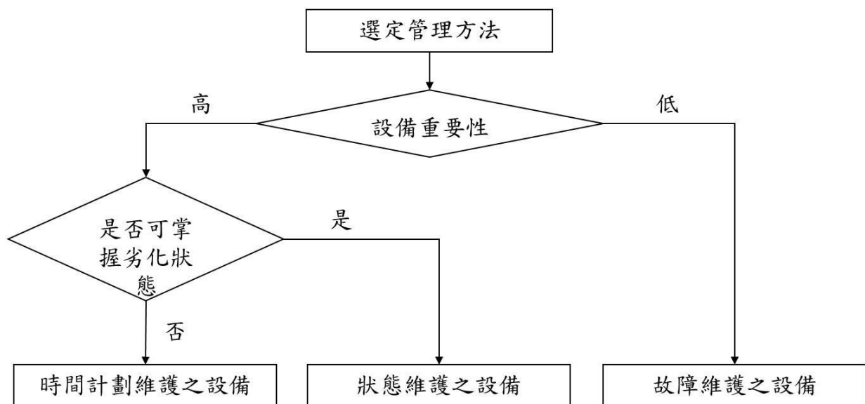
圖 6.3-2 管理方法選定流程(例)
