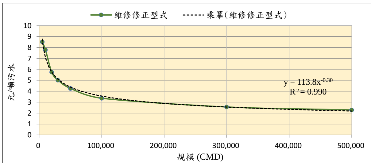
圖 2.2-3 維修修正型式之單位處理費用迴歸分析
