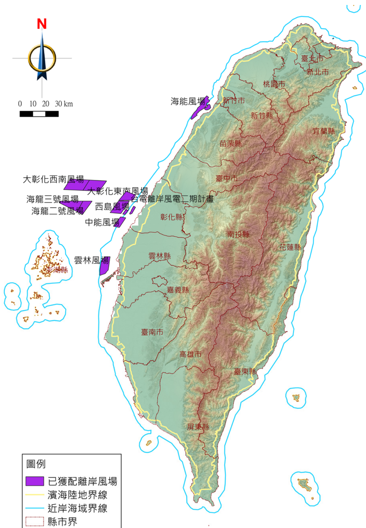
圖 2.3-2 離岸風力發電廠
