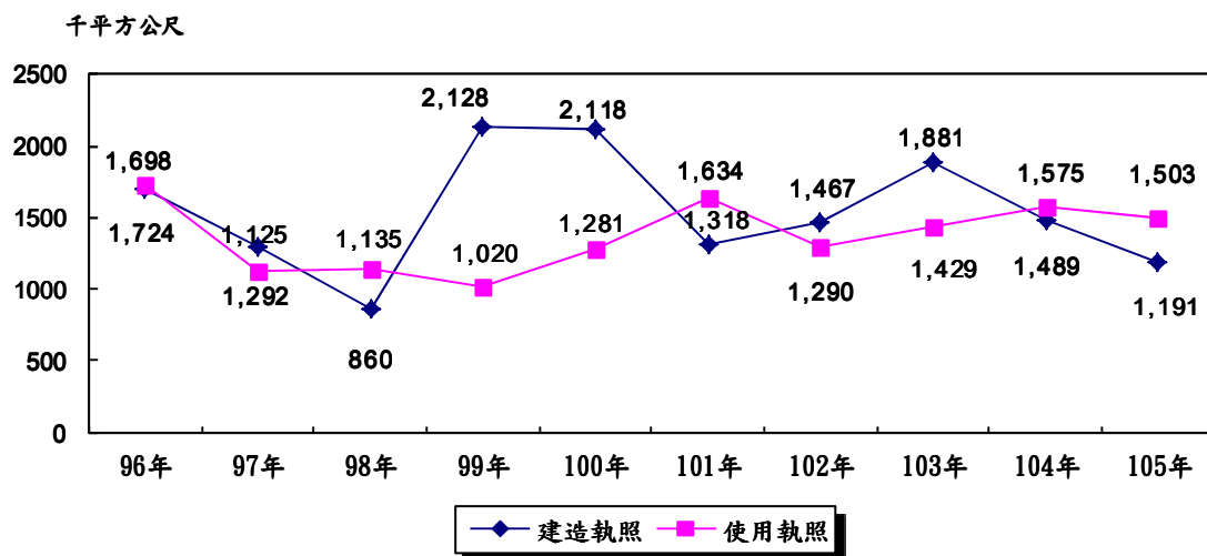
圖8 新竹縣核發建造執照及使用執照之總樓地板面積
