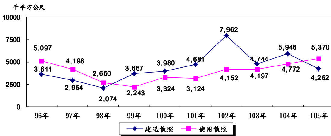
圖3 桃園市核發建造執照及使用執照之總樓地板面積
