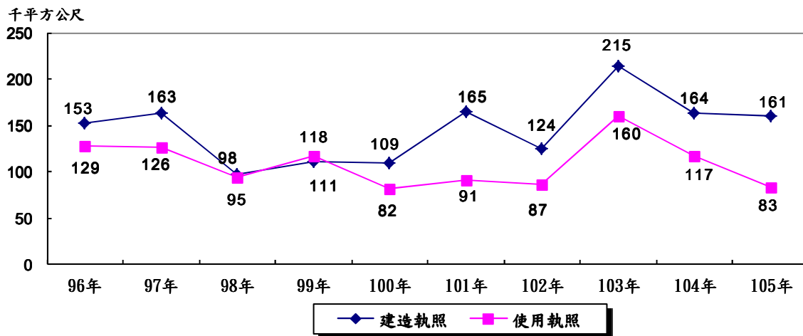
圖17 澎湖縣核發建造執照及使用執照之總樓地板面積
