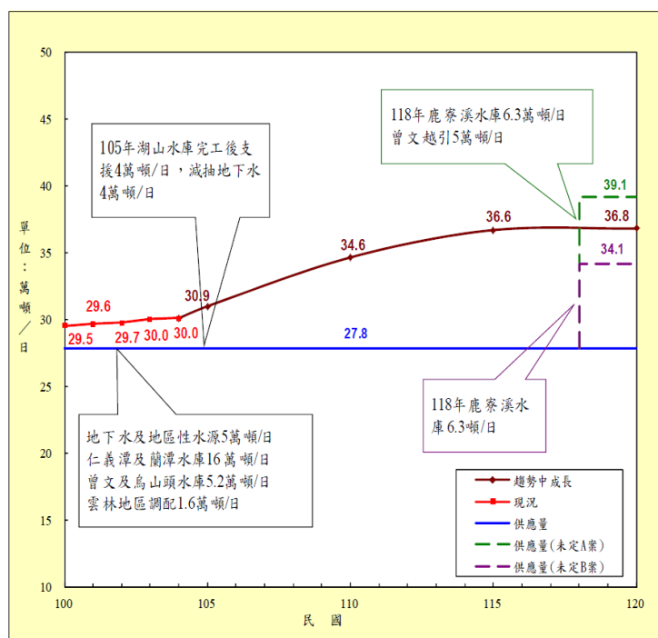
圖 2-3-3 嘉義地區生活及工業用水供需比較
