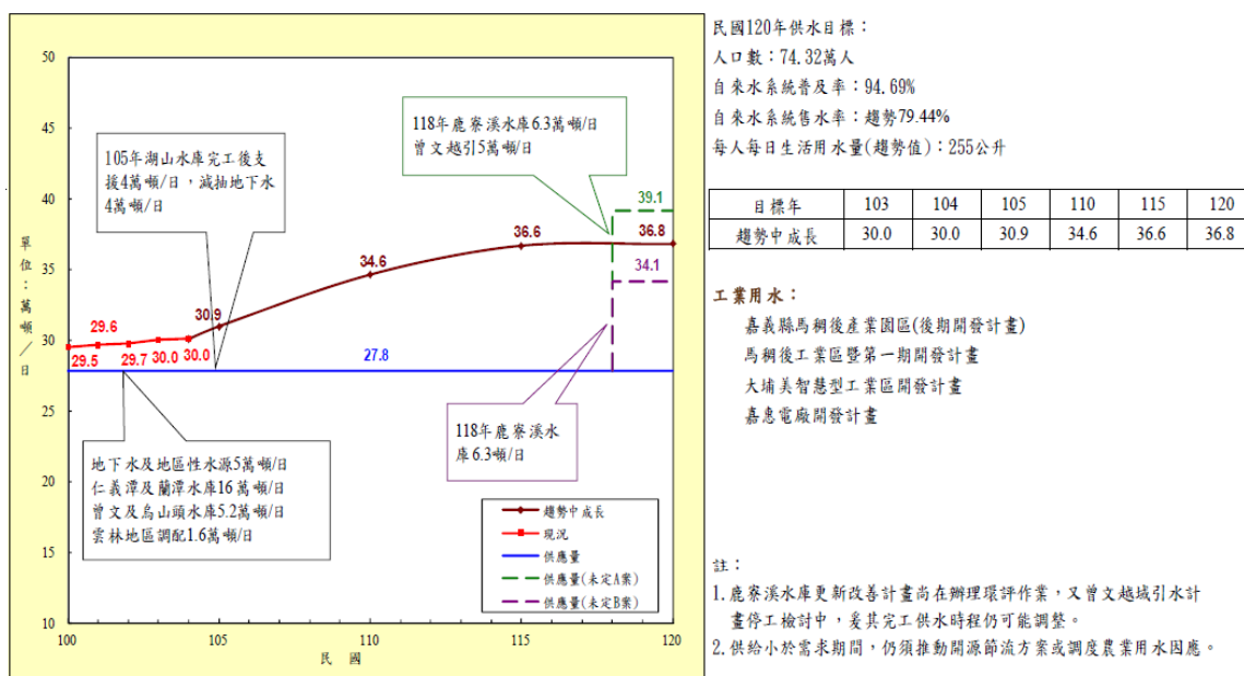
圖 5-9-5 嘉義地區自來水系統用水供需圖
