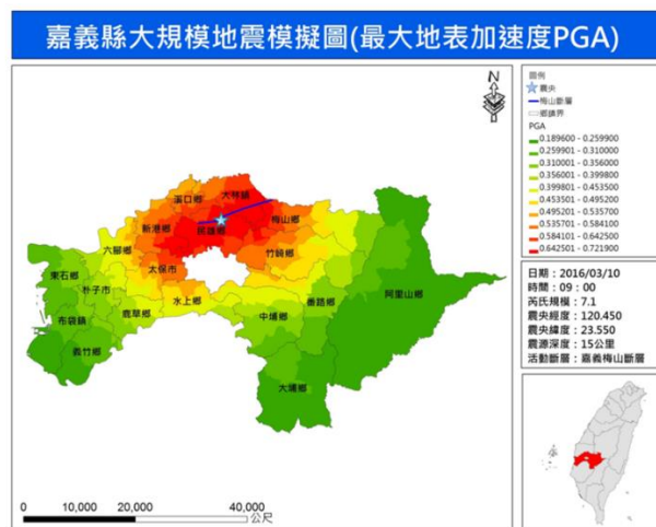
圖 5-8- 12 嘉義縣模擬梅山斷層大規模地震模擬圖(最大地表加速度PGA)
