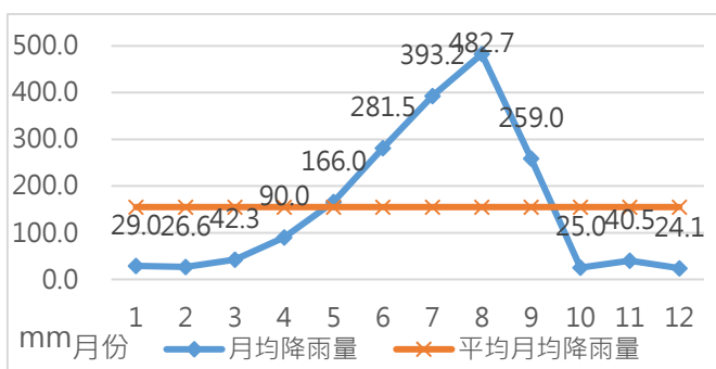
圖 2-2-7 嘉義縣月均降雨量比較圖
