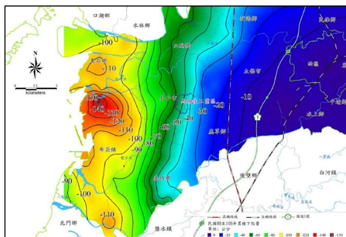
圖 2-2- 23 嘉義地區民國 80 至 106 年累積下陷量圖
