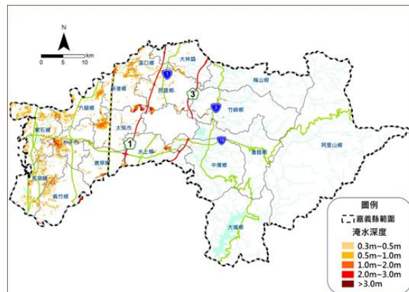
圖 5-8- 17 淹水潛勢(24 小時 350mm 降雨)
