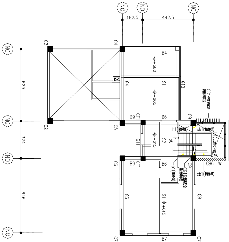
三層結構平面圖 S:1/100
