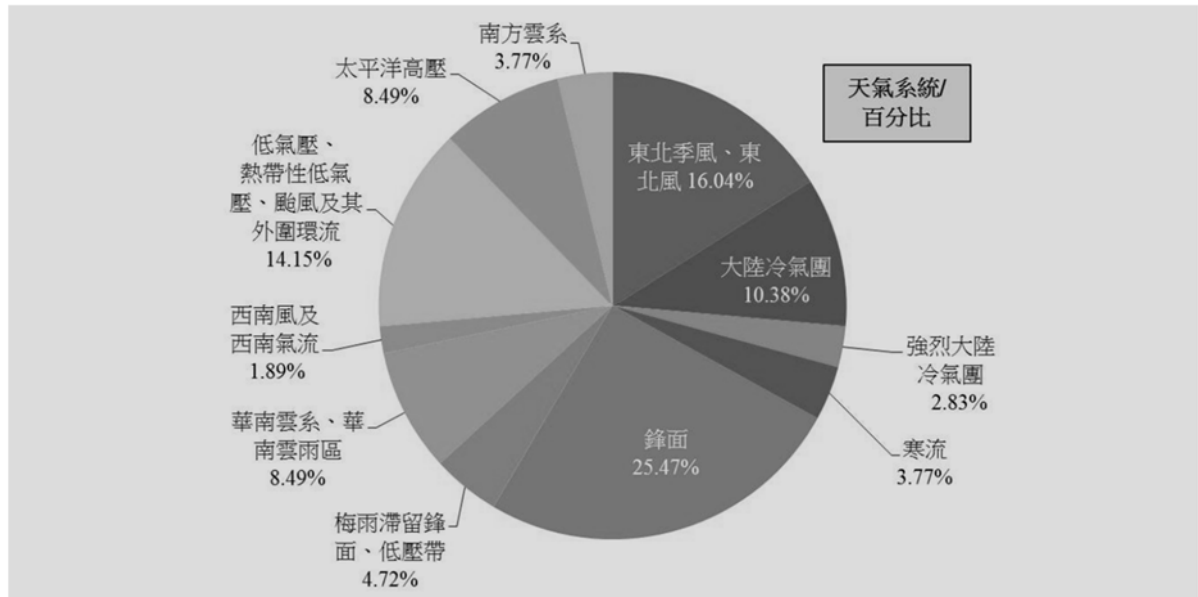
圖 2-2-4 民國 105 年影響臺灣之天氣系統比例示意圖
