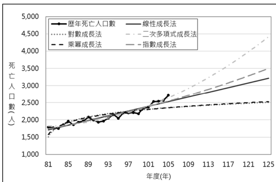
圖 3-4-2 新竹市死亡人口預測分析圖
