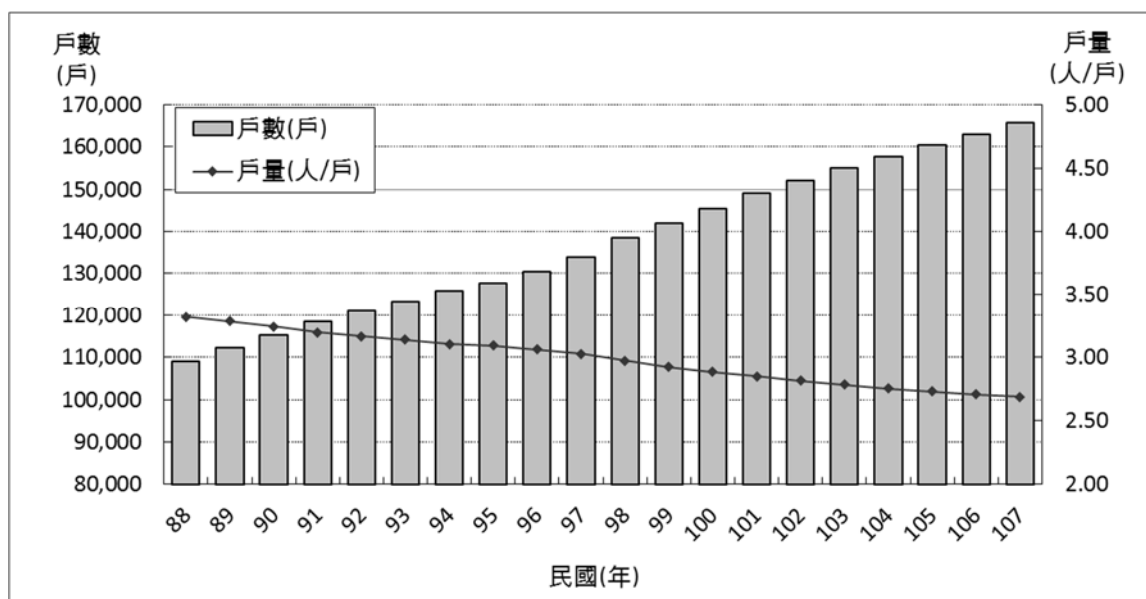
圖 2-2-32 新竹市戶數與戶量成長趨勢示意圖
