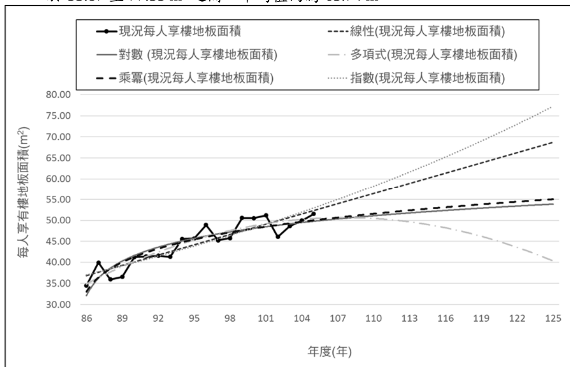
圖 3-2-1 新竹市每人享有樓地板面積預測分析圖
