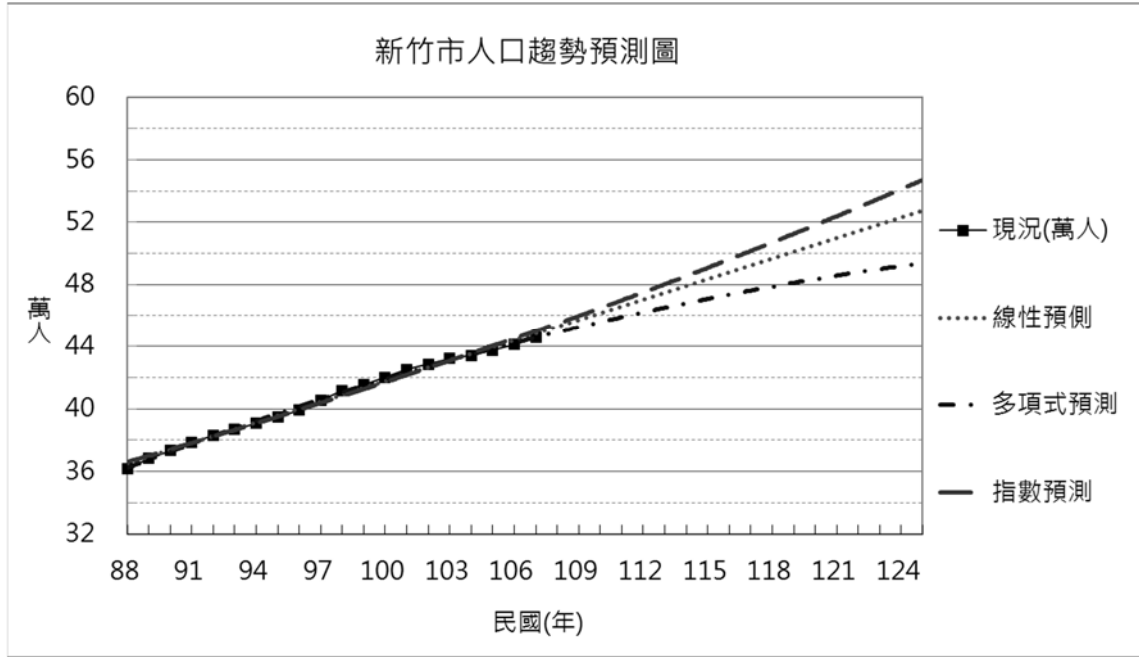
圖 3-1-1 新竹市人口預測趨勢圖
