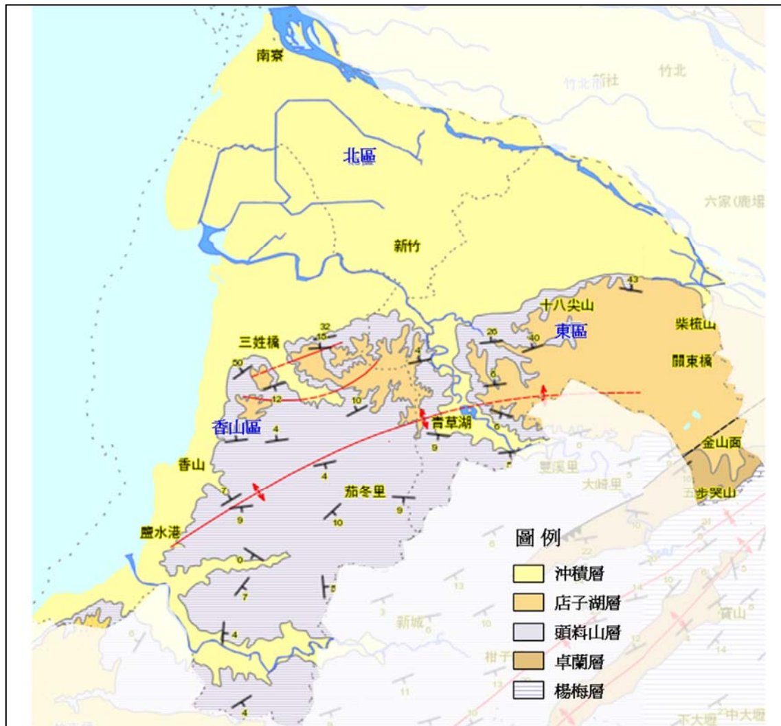
圖 2-2-2 地質分布示意圖
