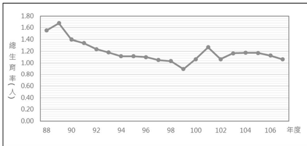
圖 3-1-3 歷年全國總生育率趨勢示意圖
