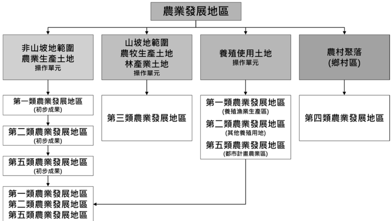
圖 6-2-3 農業發展地區分類劃設作業程序示意圖
