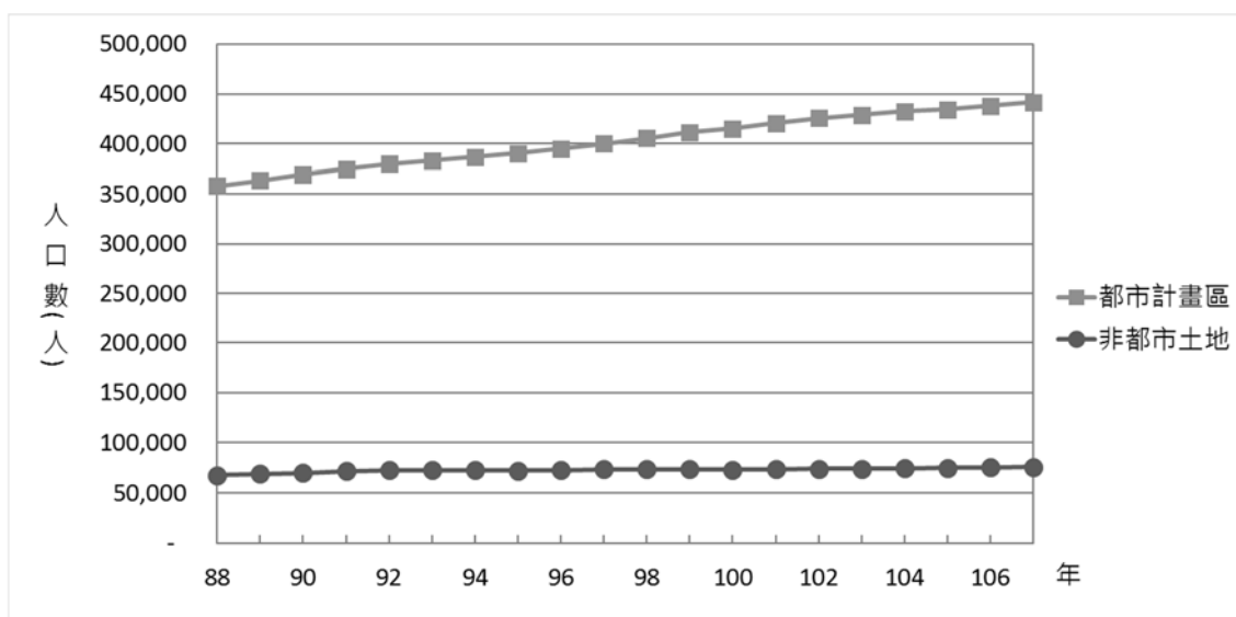
圖 2-2-29 新竹市都市計畫區與非都市土地人口成長趨勢圖
