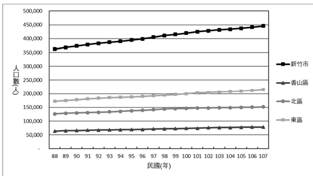
圖 2-2-28 新竹市各行政區歷年人口成長趨勢圖
