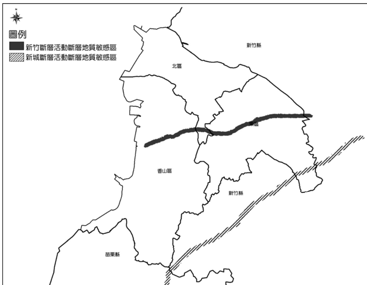
圖 2-2-3 新竹市活動斷層分布示意圖
