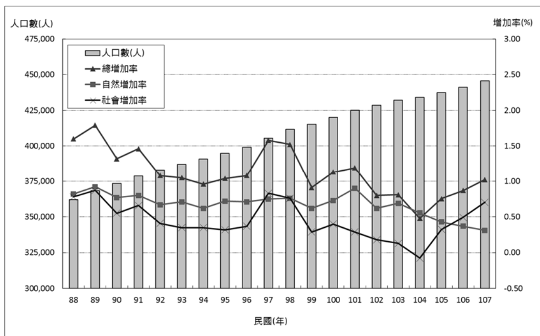
圖 2-2-27 新竹市人口動態示意圖
