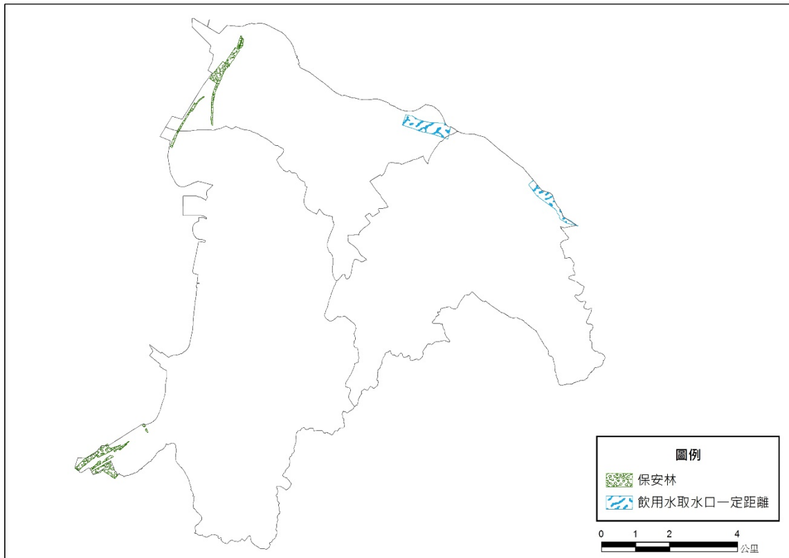
圖 2-2-19 第一級資源利用敏感地區區位分布示意圖
