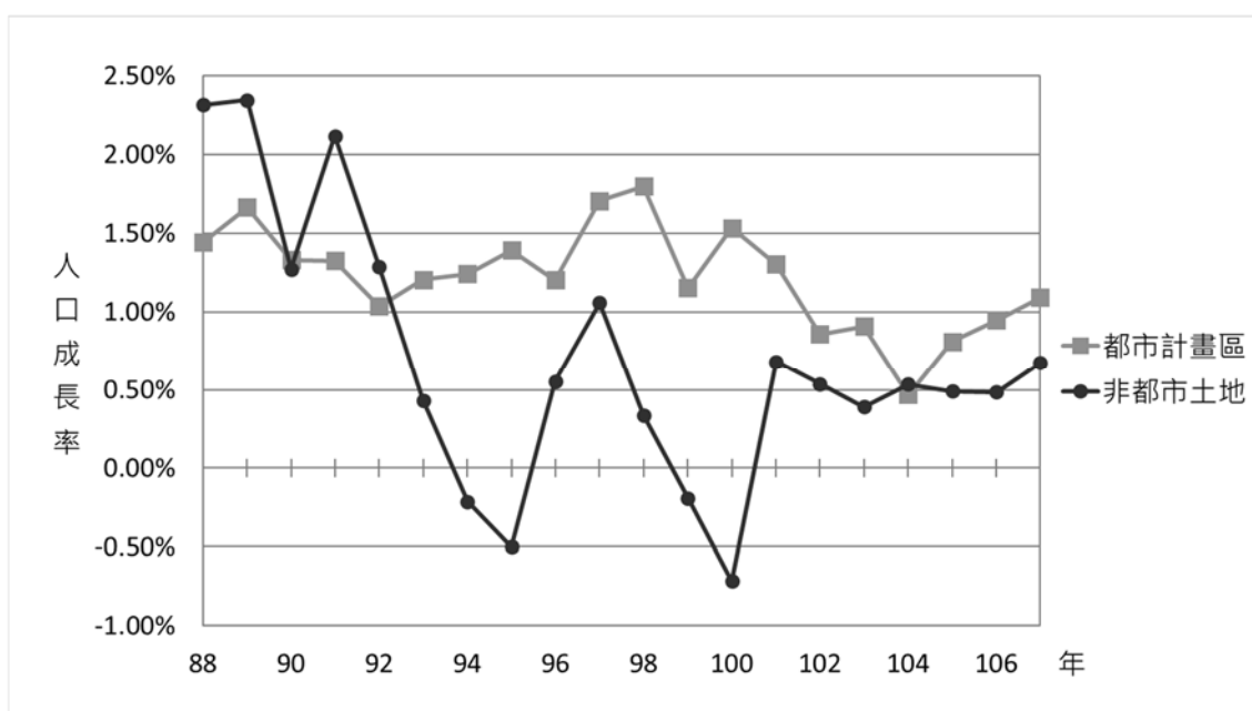
圖 2-2-30 新竹市都市計畫區與非都市土地人口年成長率折線圖
