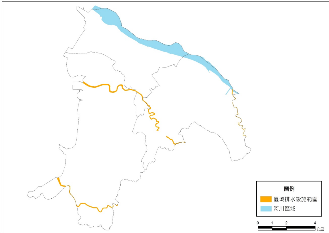
圖 2-2-13 新竹市第一級災害敏感地區區位分布示意圖
