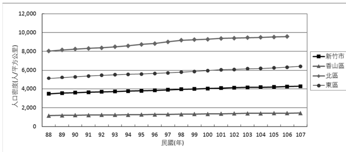
圖 2-2-31 新竹市與各行政區人口密度成長折線圖
