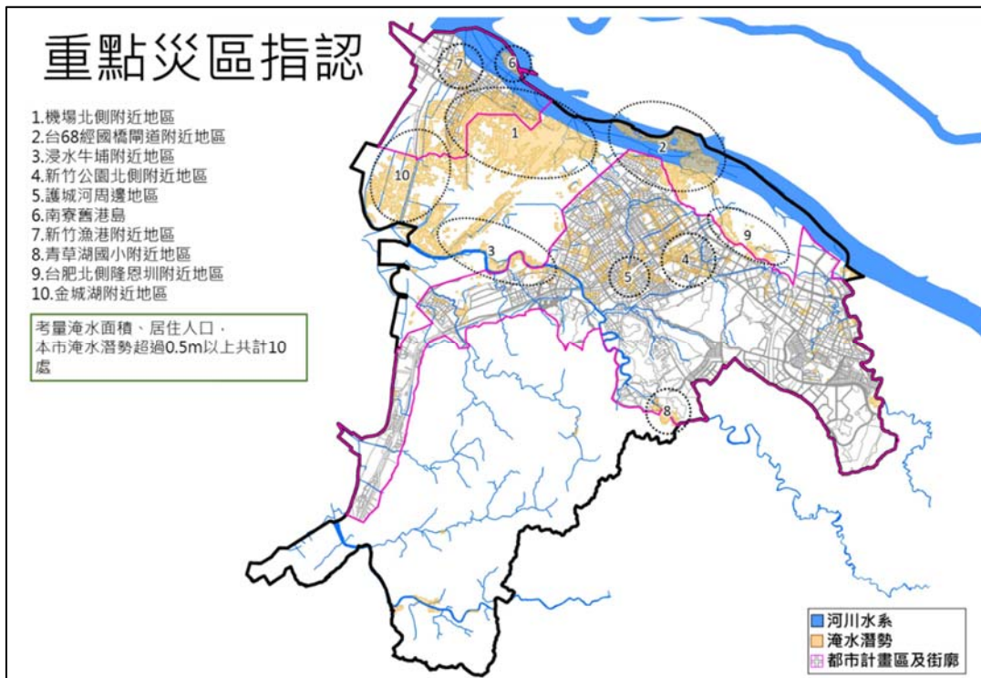
圖 8-2 新竹市颱風淹水災害重點災區指認示意圖
