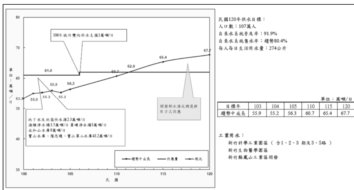
圖 3-4-3 經濟部水利署推估 120 年用水系統供需示意圖
