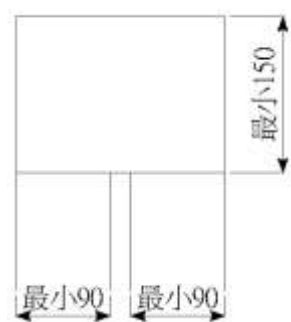
圖 206.3.3.2 坡道迴轉
