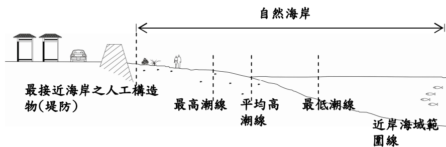
自然海岸剖面示意圖(B)
