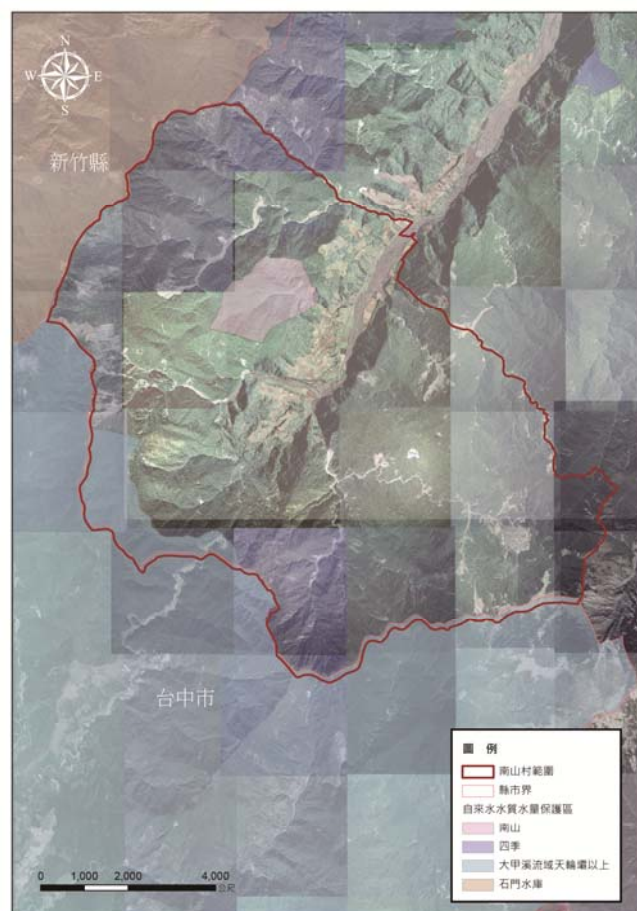
圖 3-4- 8 南山村境內及鄰近自來水水質水量保護區分佈圖
