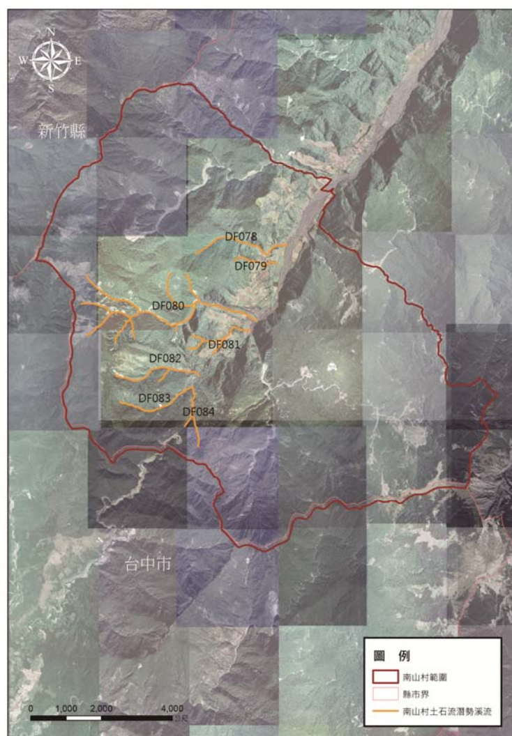
圖 3-4- 7 南山村境內土石流潛勢溪流分佈圖
