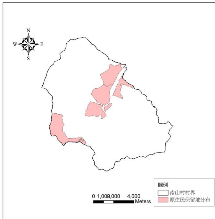
圖 3-1-2 南山村原住民保留地分布圖
