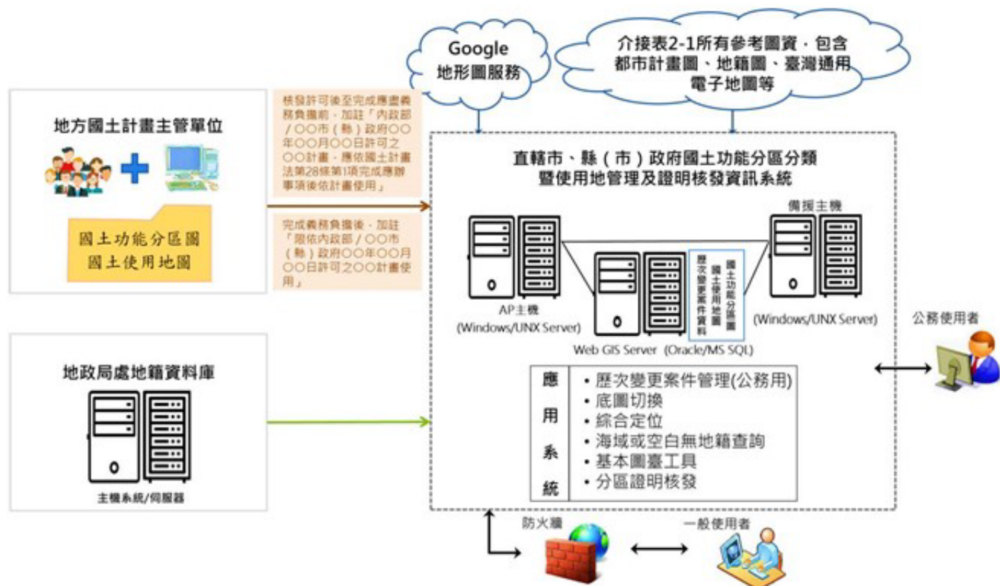
圖13 地方版系統架構圖
