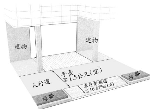
斜視圖
