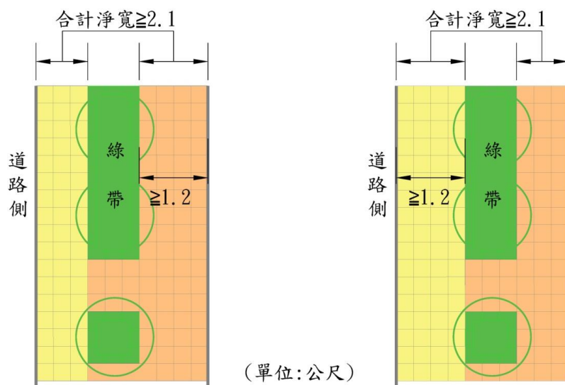
圖 6.1.1 綠帶位於人行道中央參考圖
