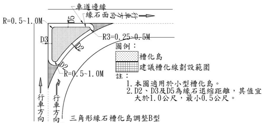
圖 C4.18.1 三角形槽化島佈設原則及設計型式參考圖例
