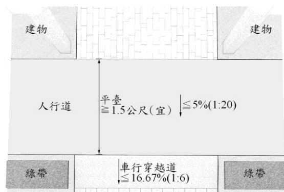
平面圖
