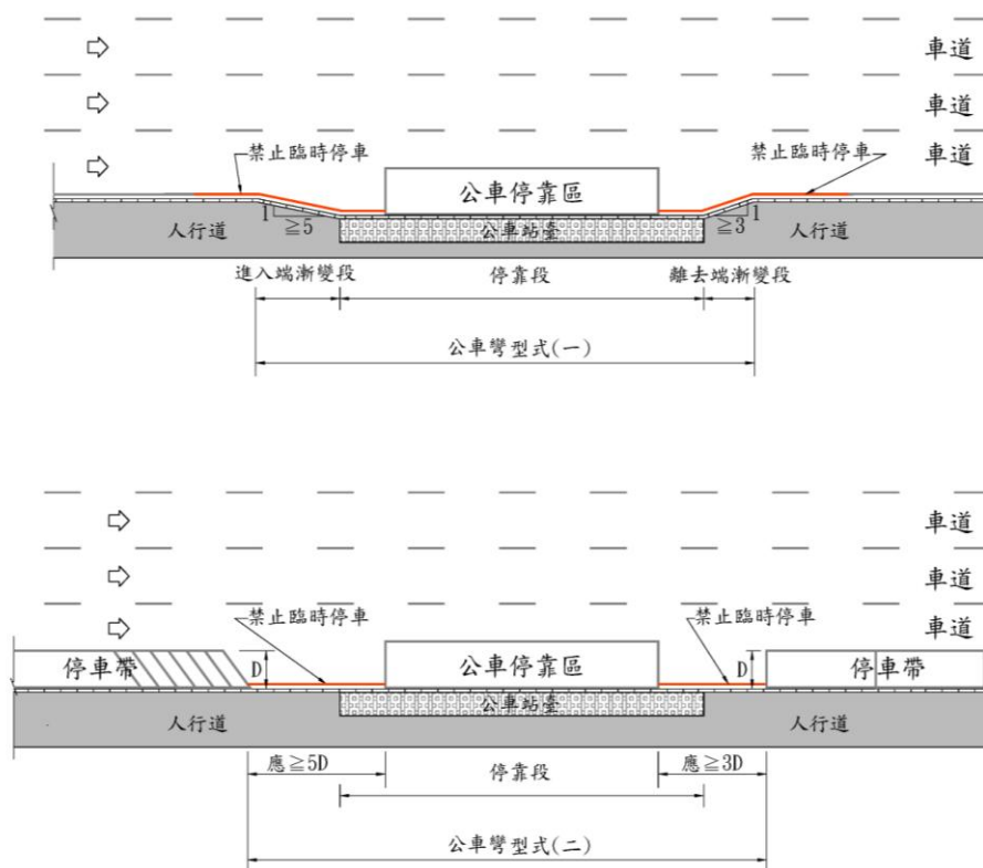
圖 10.1.2 公車彎設置參考圖
