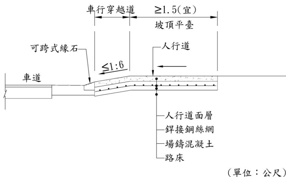
圖 6.3.4 車行穿越道搭配可跨式緣石斷面配置參考圖
