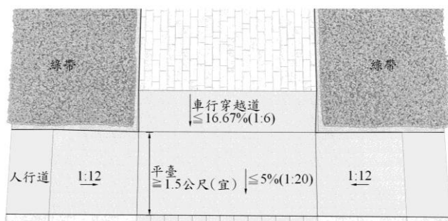
平面圖
