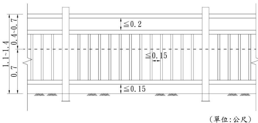
圖 6.6.3 行人欄杆桿件最大淨距參考圖
