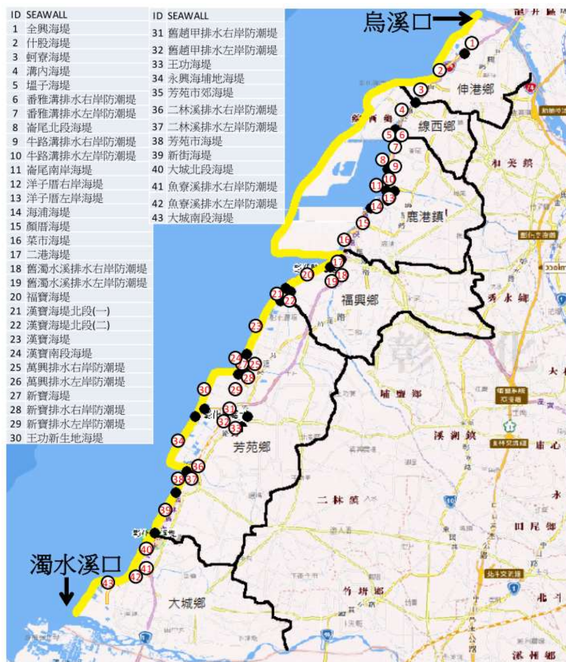
圖 2-2 彰化縣海堤設施位置圖
