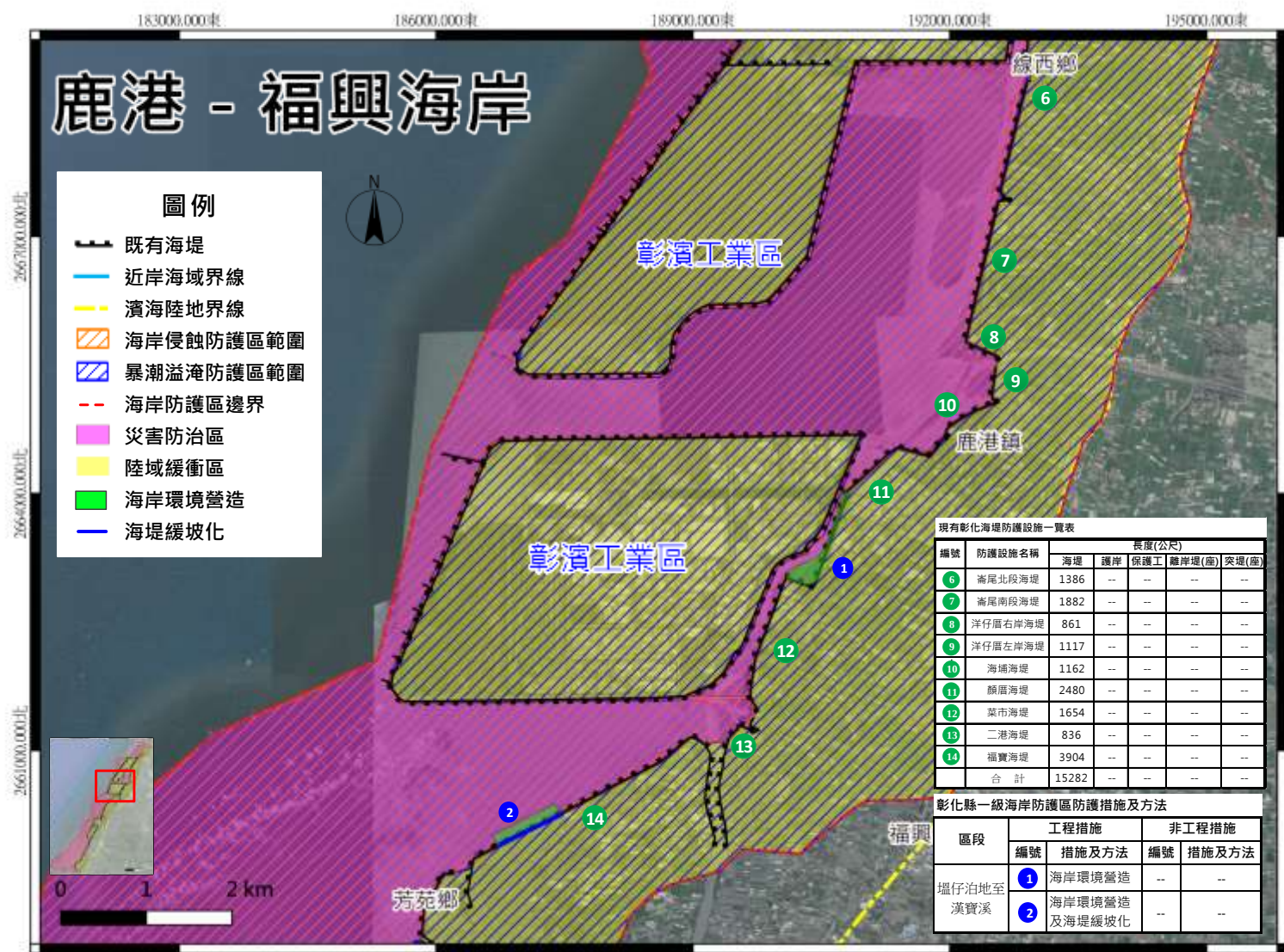
圖 7-3 塭仔泊地至漢寶溪海岸防護設施種類、規模及配置圖
