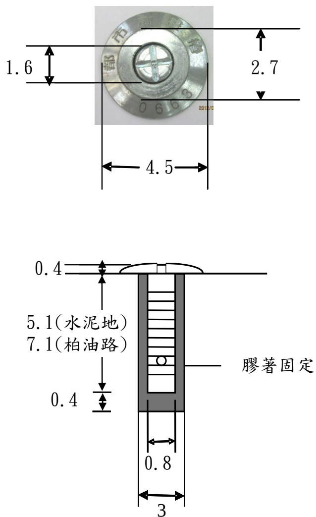
附圖二 都市計畫樁埋設規格（含泥土地）
