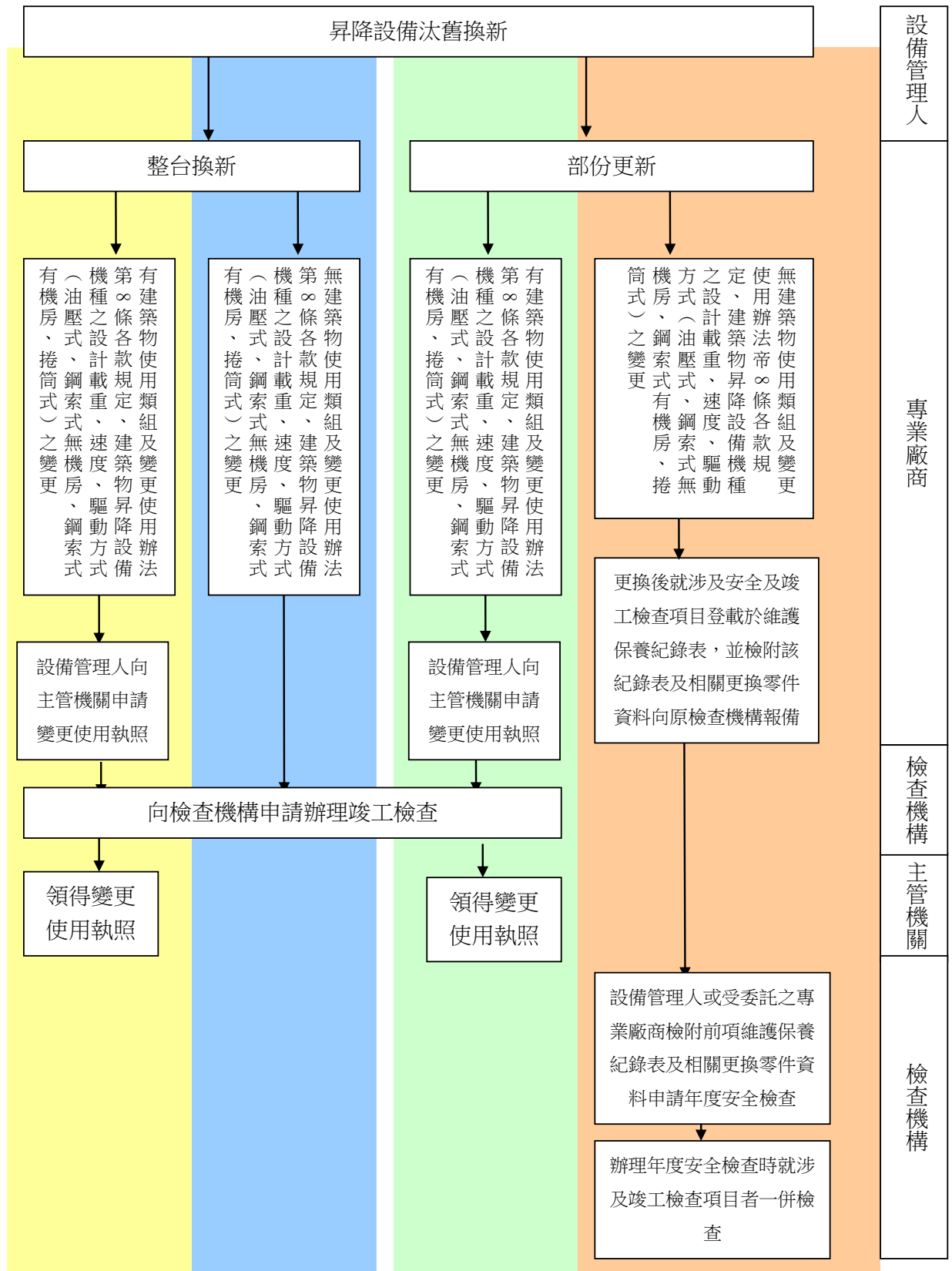
建築物昇降設備汰舊換新流程圖
