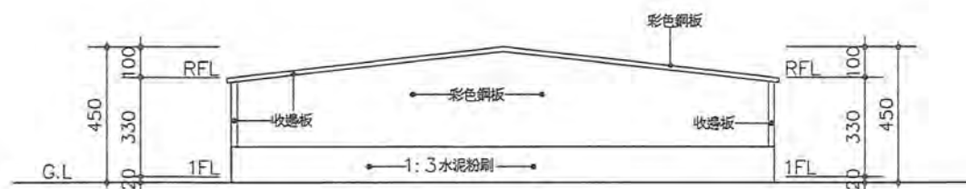
(北向) 左側立面圖 S=1:150
