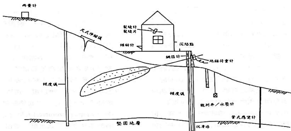
圖 2-11 山坡地安全觀測系統配置示意圖
