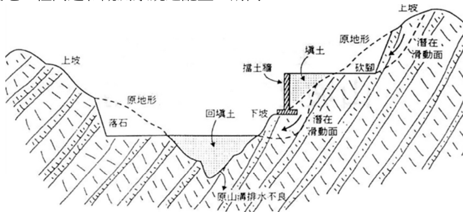
圖 2-10 山坡地工程可能引發之坡地問題
