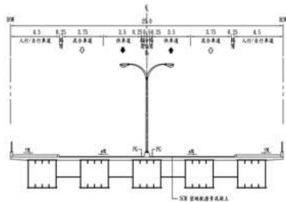
↑ 橋梁橫斷面圖（南工處提供）
