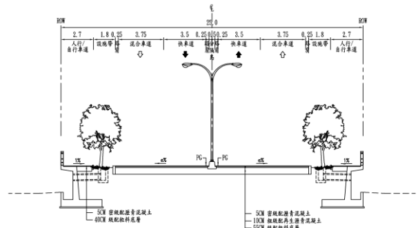
↑ 道路橫斷面圖（南工處提供）
