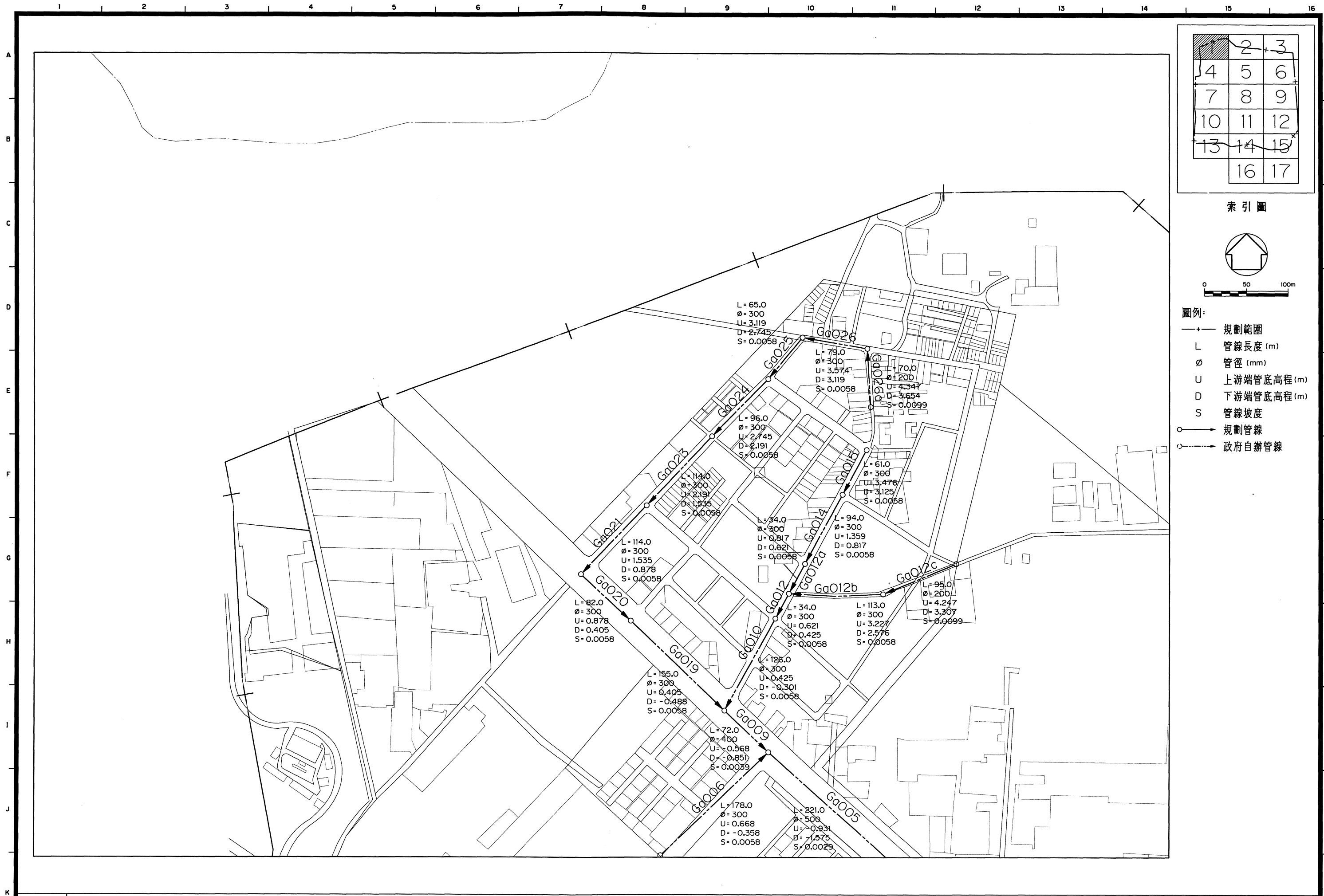
圖 4.5-4 岡山地區污水下水道系統平面配置圖(1/17)
