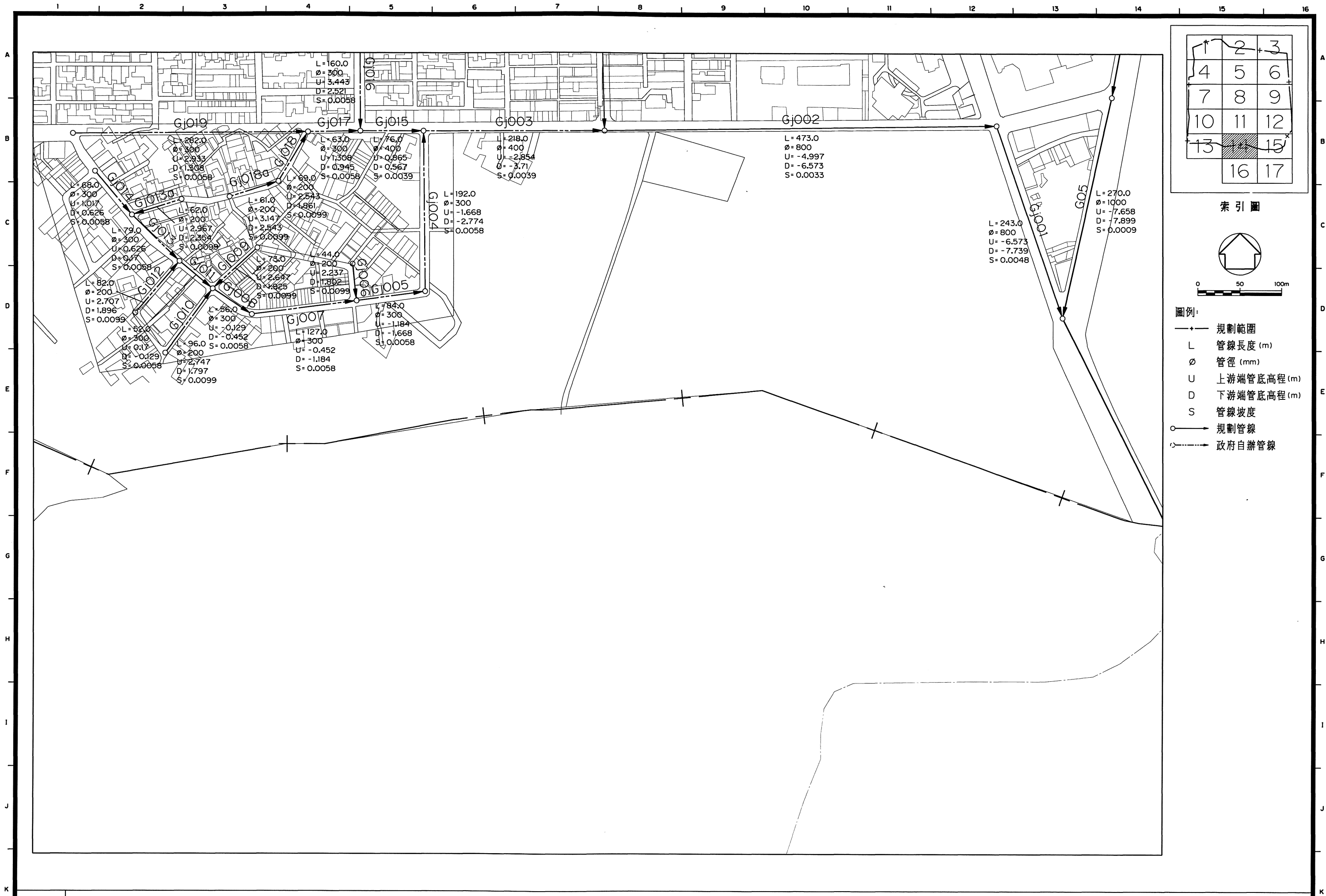
圖 4.5-4 岡山地區污水下水道系統平面配置圖(14/17)
