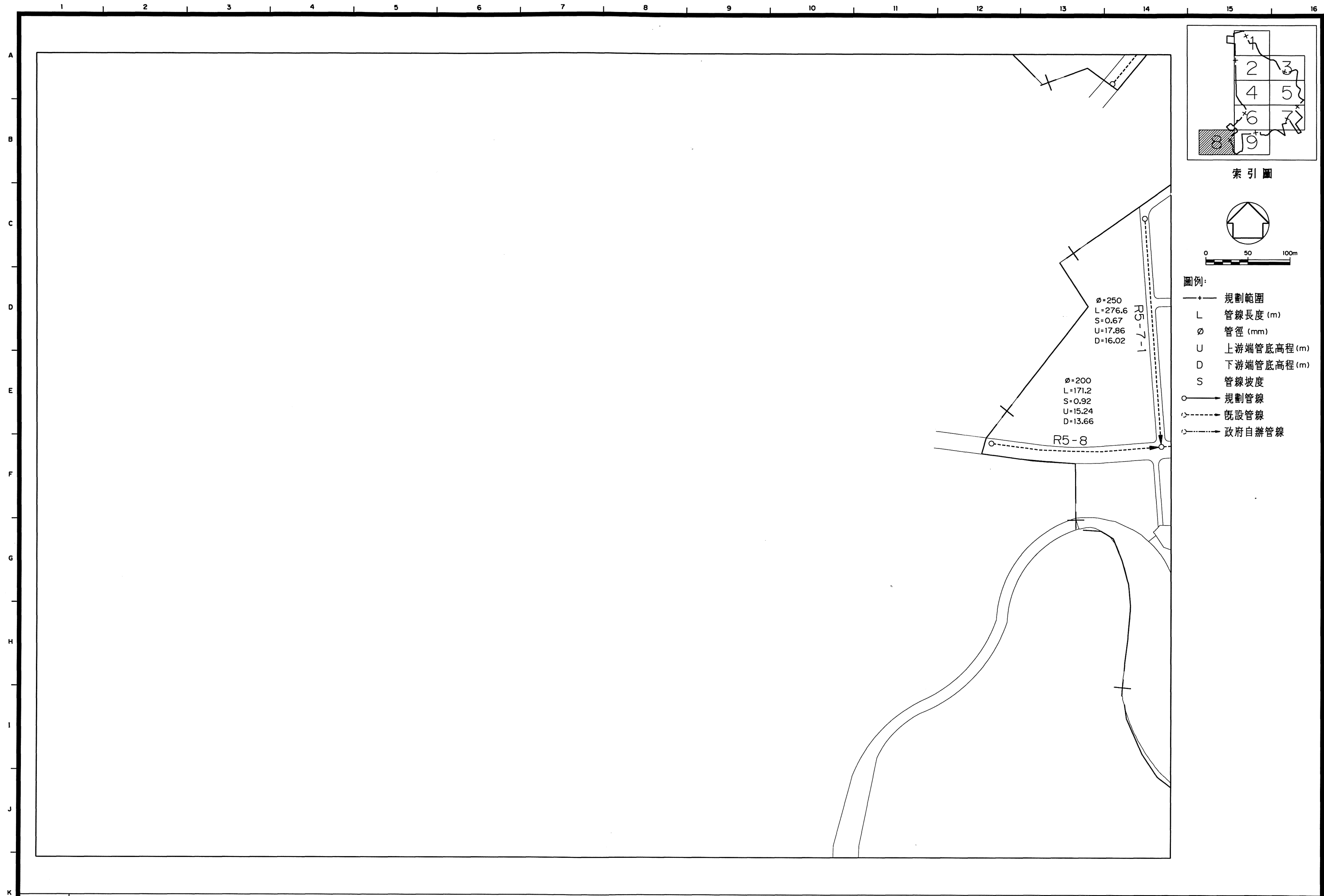
圖4.3.4-4 橋頭地區污水下水道系統平面配置圖(8/9)
