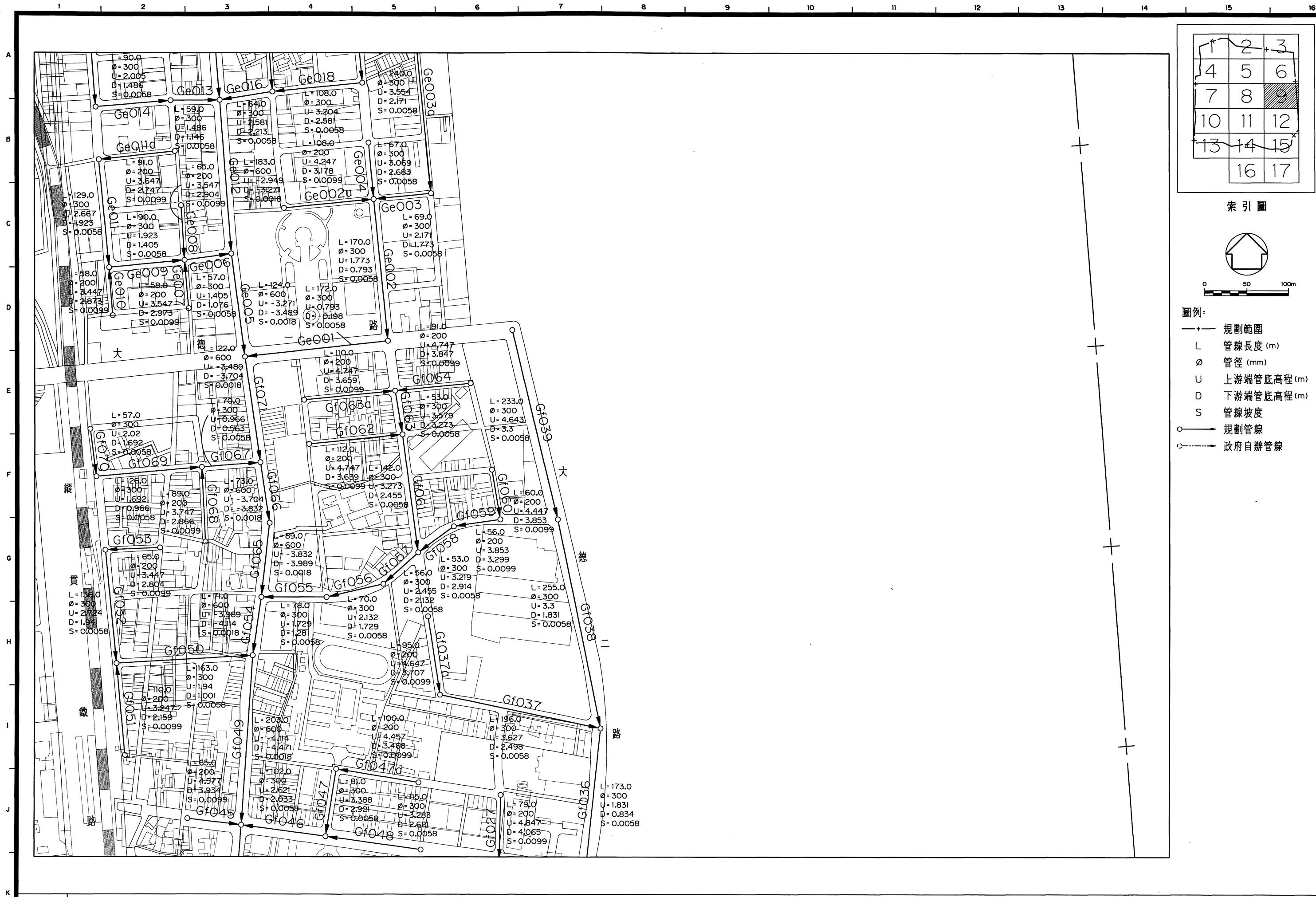
圖 4.5-4 岡山地區污水下水道系統平面配置圖 (9/17)
