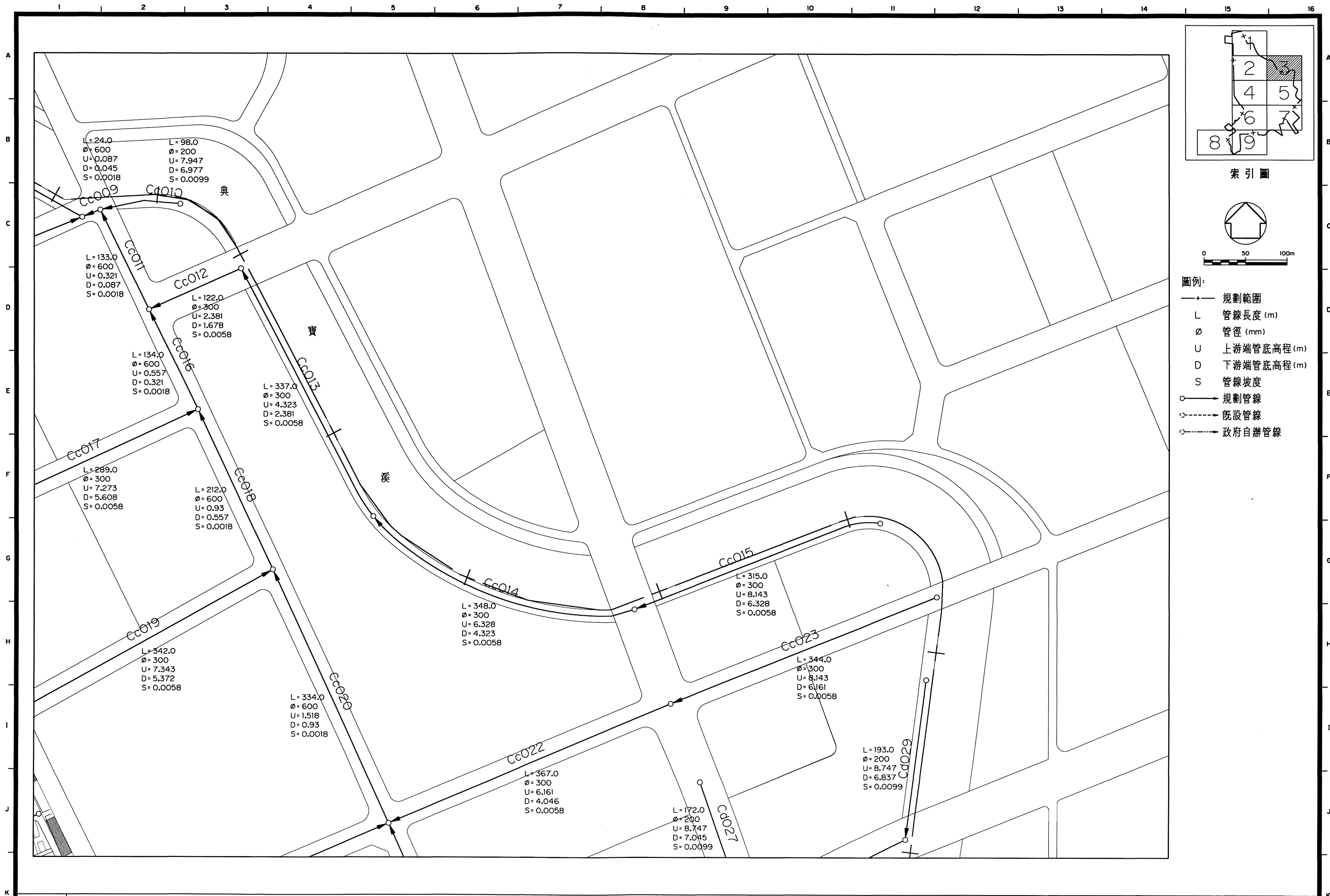
圖 4.3.4-4 橋頭地區污水下水道系統平面配置圖(3/9)
