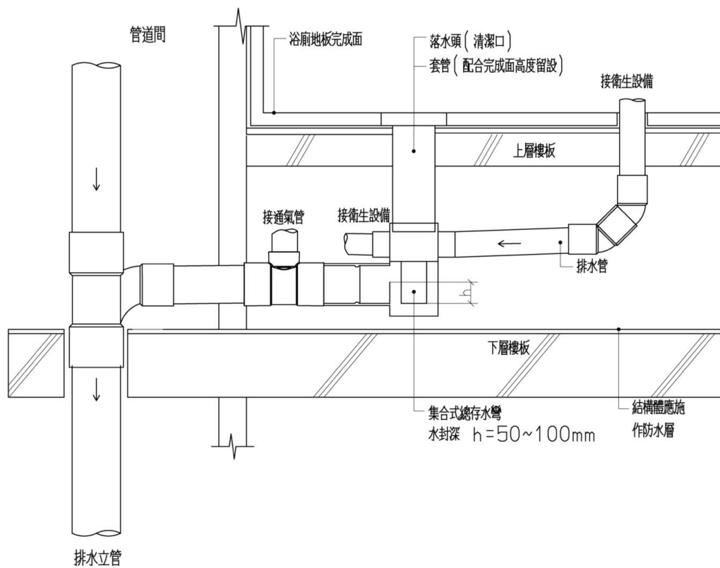
圖4-18-3 同層降板式（雙層樓板）剖面示意圖
