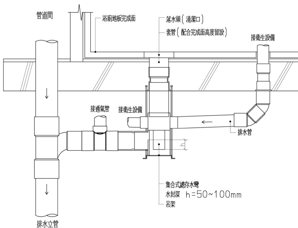
圖4-18-4 隔層懸吊式剖面示意圖
