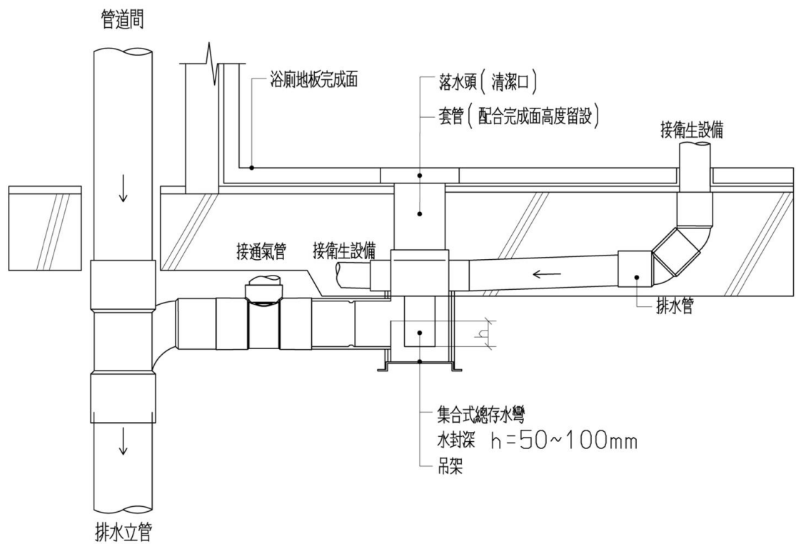
圖4-18-5 隔層半埋入式剖面示意圖
