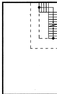
直通樓梯例(二) 虛線範圍表示樓梯間
