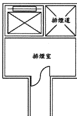
雙向甲種防火門例(一)
