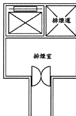
雙向甲種防火門例(二)
