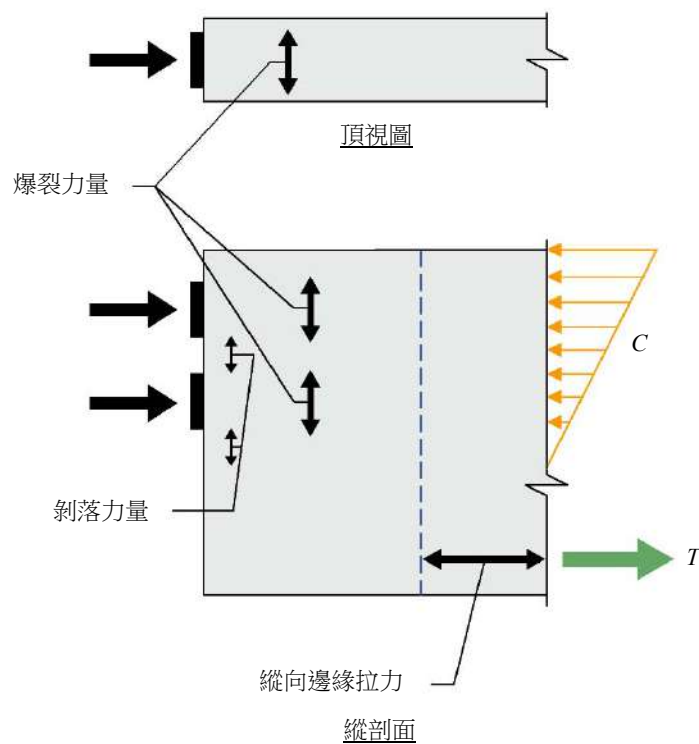
圖R25.9.4 一般區域內之拉應力區
