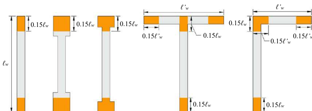
圖R18.7.2.4 第18.7.2.4(a)節所需縱向鋼筋在不同牆斷面形狀時之配置區域
