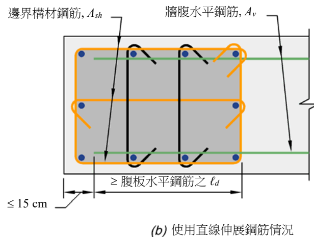
圖R18.7.6.4c 牆體水平鋼筋在受圍束之邊界構材中的伸展
