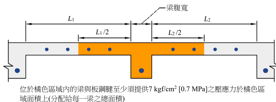
圖R7.6.4.2 梁板一體澆置之斷面
