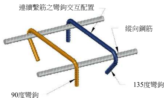
圖R25.3.5 繫筋
