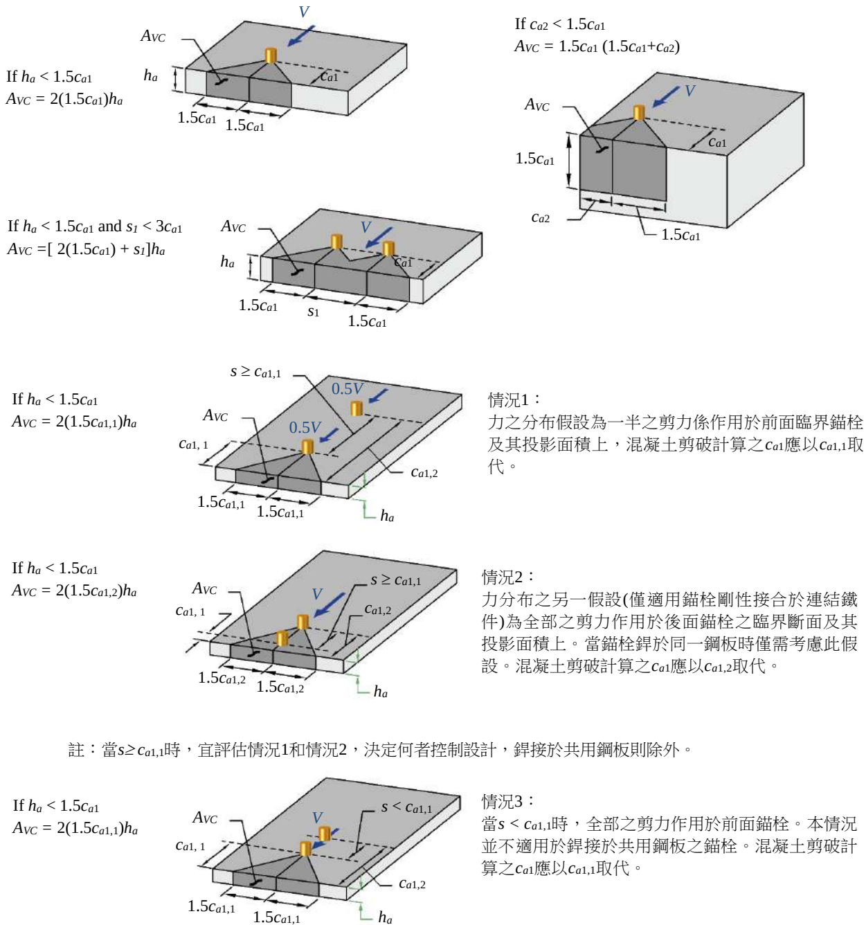
圖R17.7.2.1b 單根錨栓及錨栓群 A_{vc} 之計算
