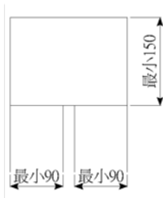
圖206.3.3.2 坡道迴轉
