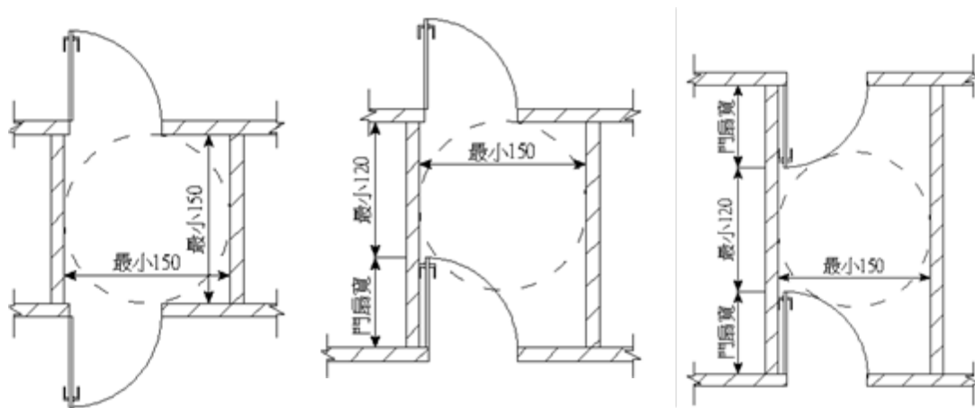
圖205.2. 4 .4 風除室所需之操作空間
