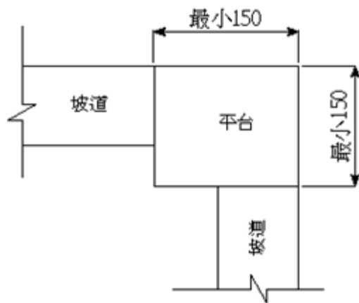
圖206.3.3.1 坡道90°轉彎
