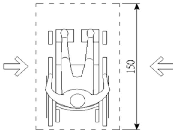
由左右側進入 圖703.2.2
