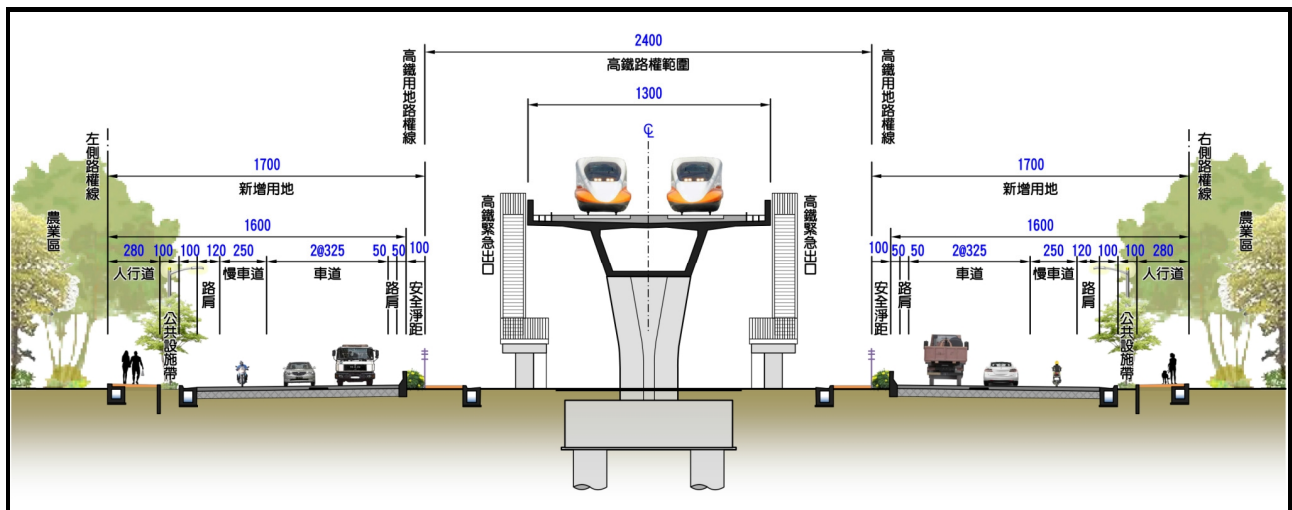
圖 15 緊鄰高鐵機房、逃生梯路段橫斷面示意圖
