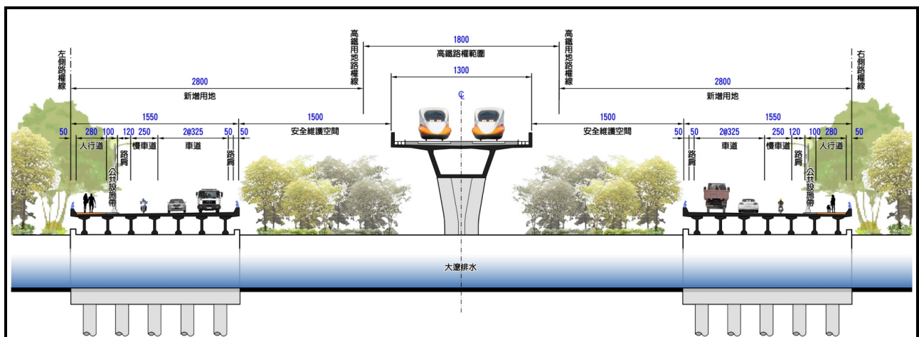
圖 16 跨河路段(PCI 樑方案)橫斷面示意圖
