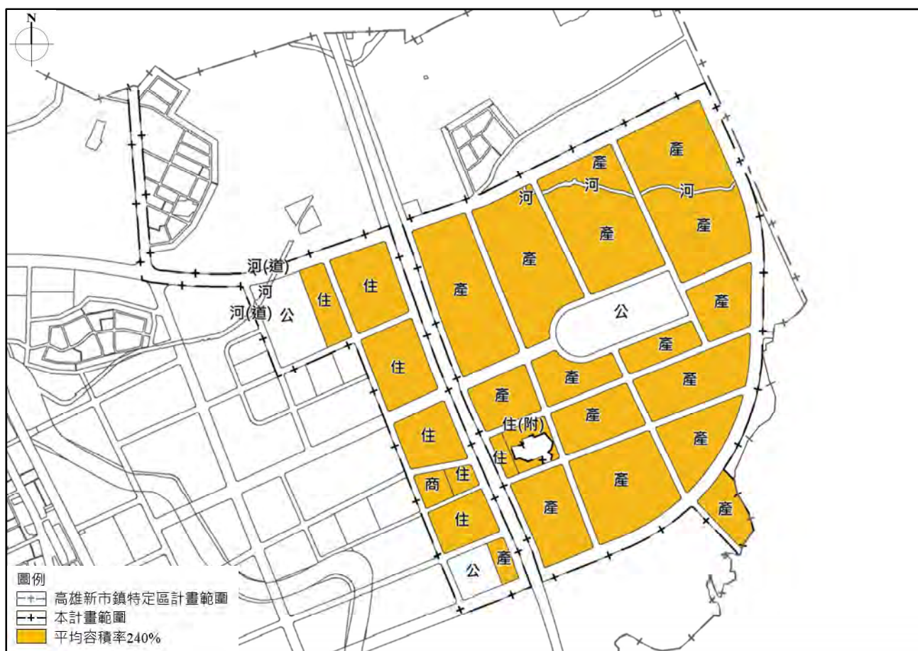
圖 2-6-1 密度管制計畫示意圖
