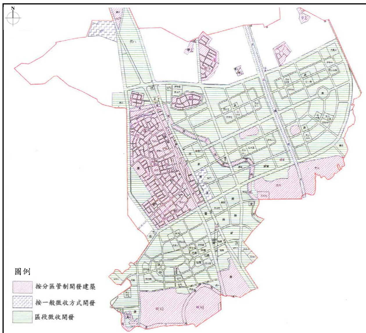
圖 2-4-2 原計畫開發方式示意圖
