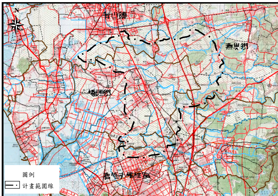
圖 4-1-1 地形示意圖
