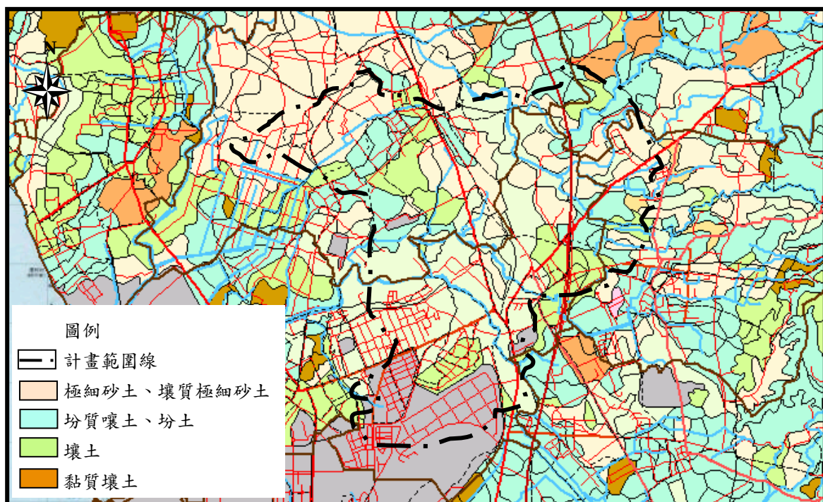
圖 4-1-3 土壤示意圖
