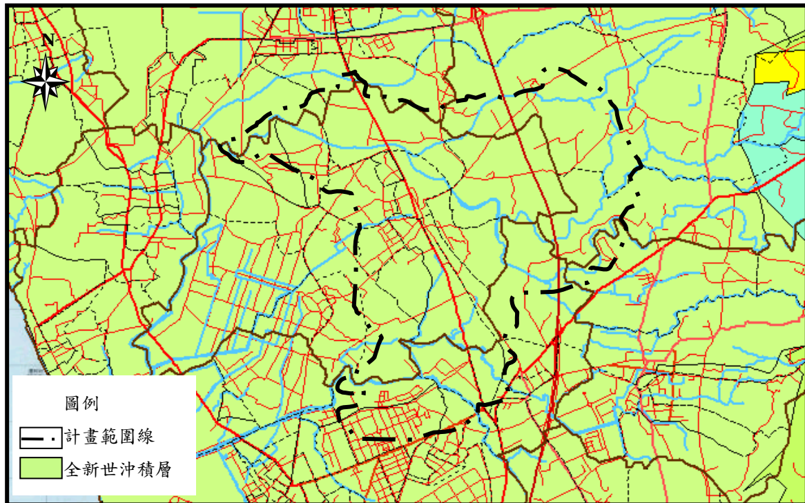
圖 4-1-2 地質示意圖
